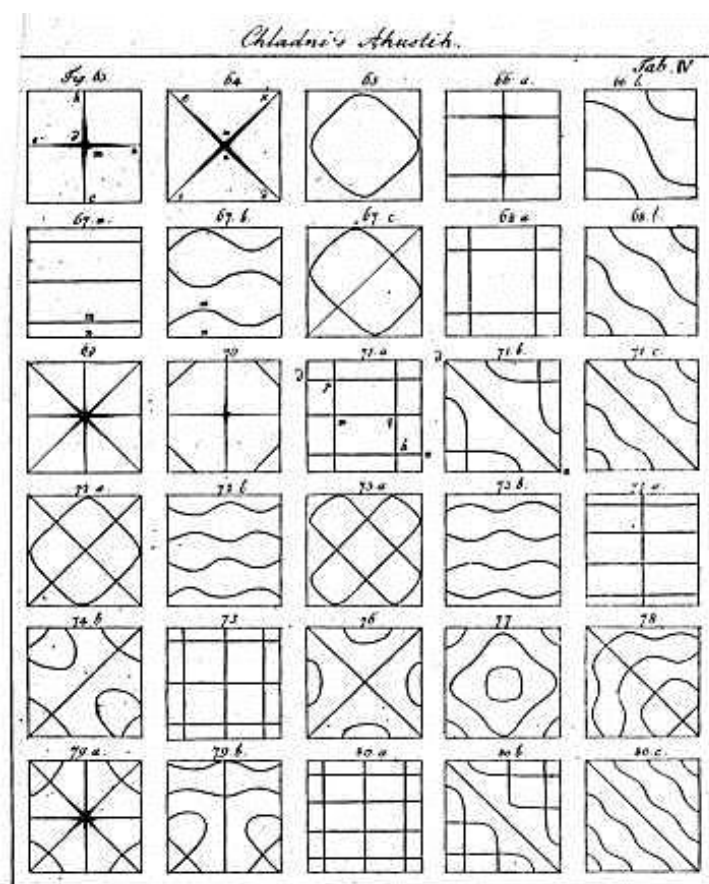
Obr. 3.2 Chladniho obrazce [5].
