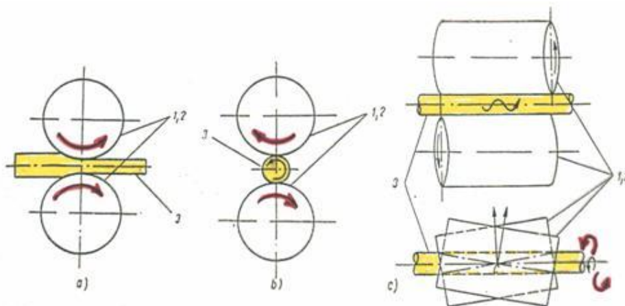
Obr. 6.1 Válcování polotovarů [45].
