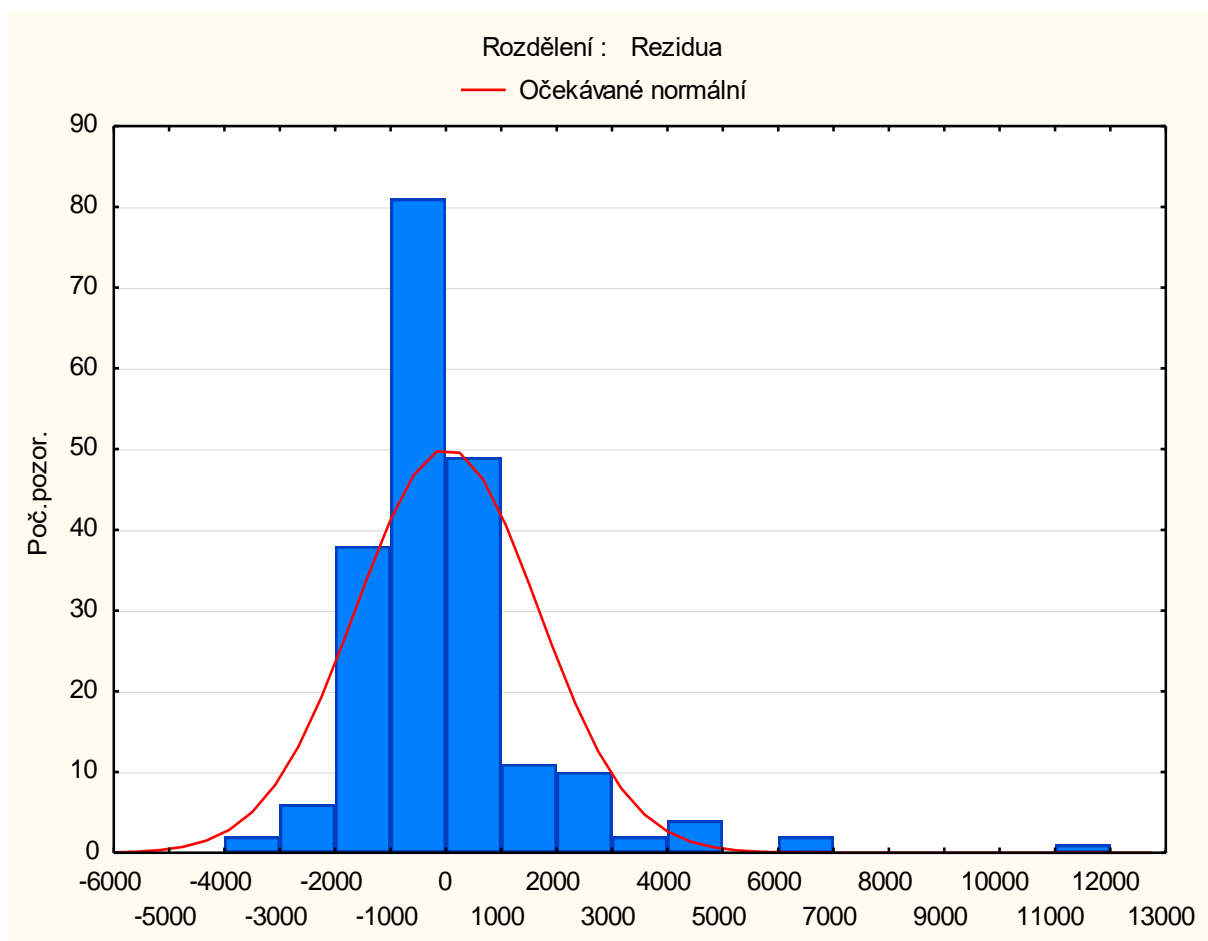
Obrázek 4.1 – Histogram reziduí
