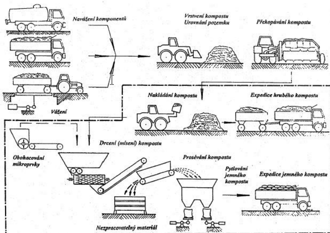
Obrázek 2.3 – Schéma kompostárny [20]
