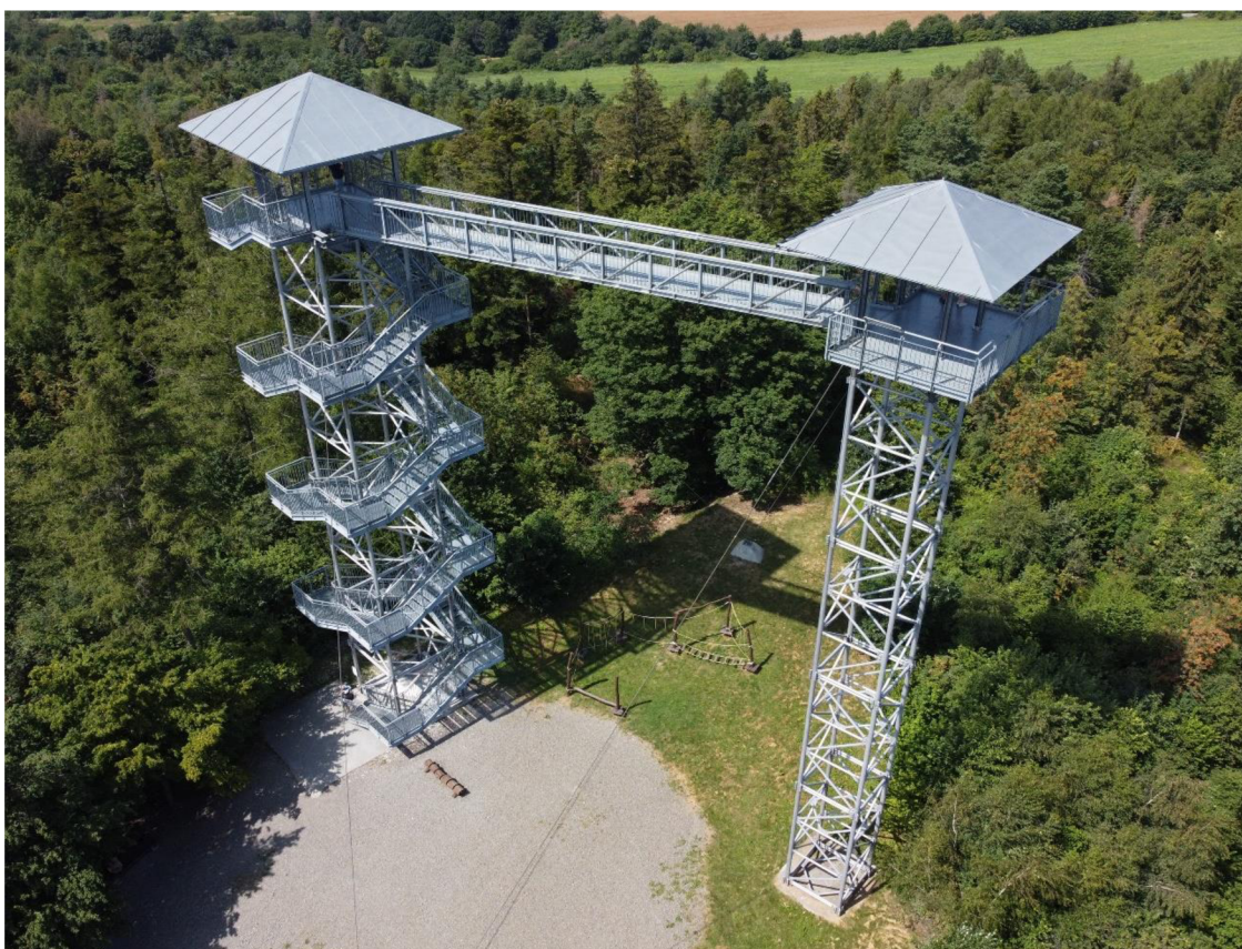
Obrázek 6.2 – Konstrukce rozhledny [39]
