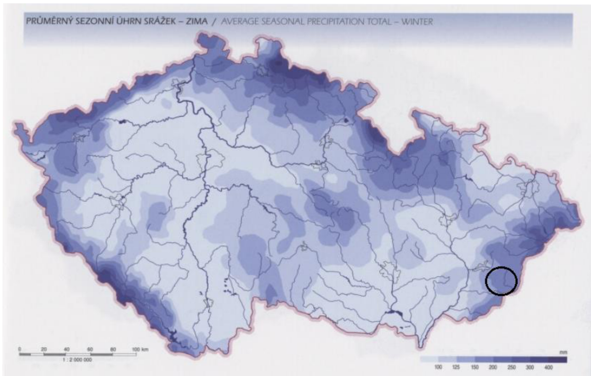
Obr. 33. Průměrný sezonní úhrn srážek – zima (převzato: TOLASZ, Radim. Atlas podnebí Česka: Climate atlas of Czechia . Praha: Český hydrometeorologický ústav, 2007. ISBN 978-80-244-1626-7., str. 71, upraveno autorka)
