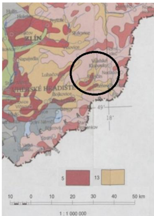
Obr. 34. Půdní mapa České republiky: 5. hnědozemě, 13. hnědé půdy se surovými půdami (převzato: TOMÁŠEK, Milan. Půdy České republiky . 4. vyd. Praha: Česká geologická služba, 2007. ISBN isbn80-7075-688-8., mapa, upraveno autorka)
