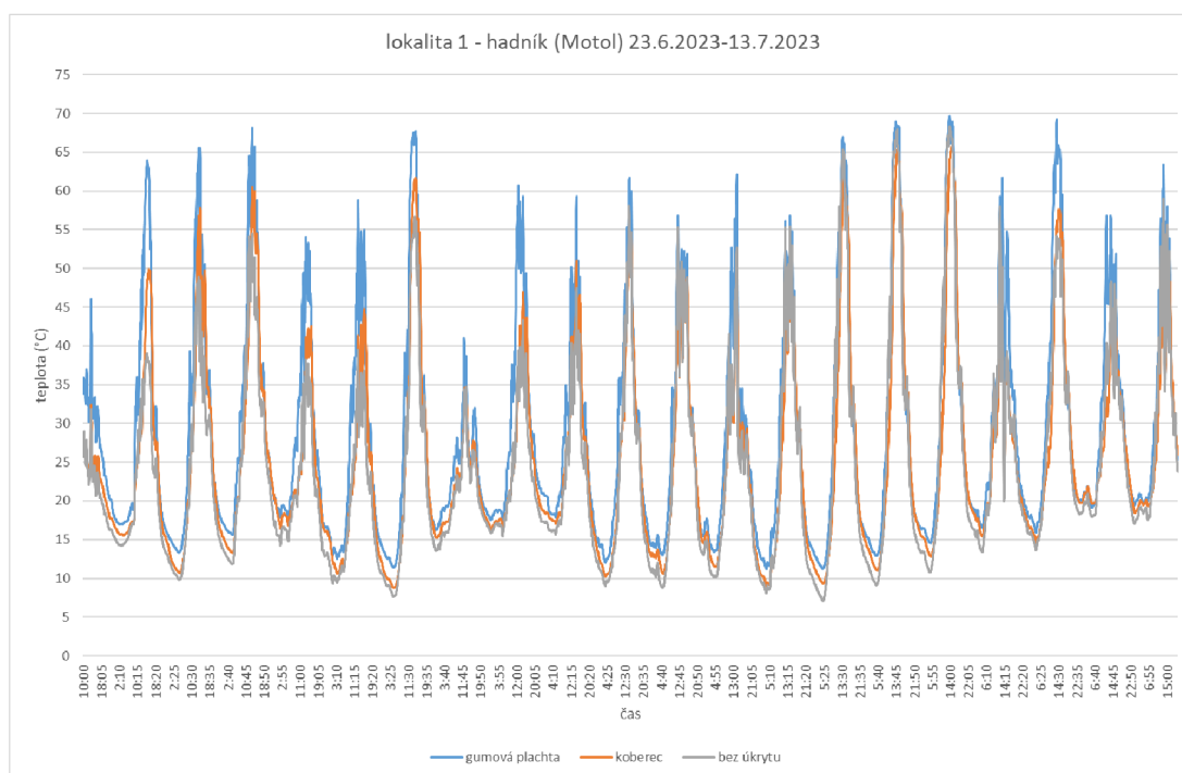
Figure 2: Lokalita 1 průběh teplot od konce června do poloviny července (data: HOBO Pendant UA-002 upravil: autor práce)
