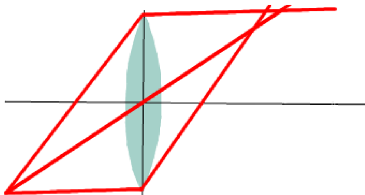
Obr. 2.7 Asymetrická vada
