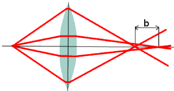
Obr. 2.6 Otvorová vada
