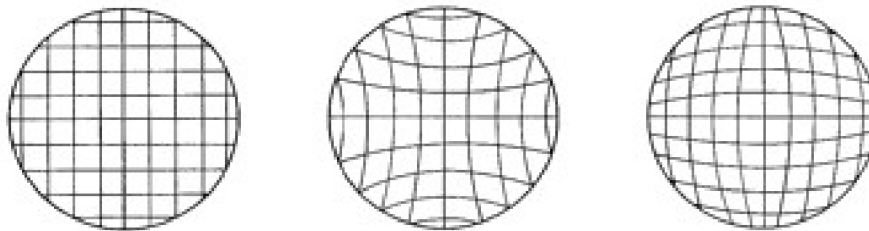
Obr. 2.9 Zkreslení obrazu (nezkraslený, poduškovité, soudkovité), převzato z [4]
