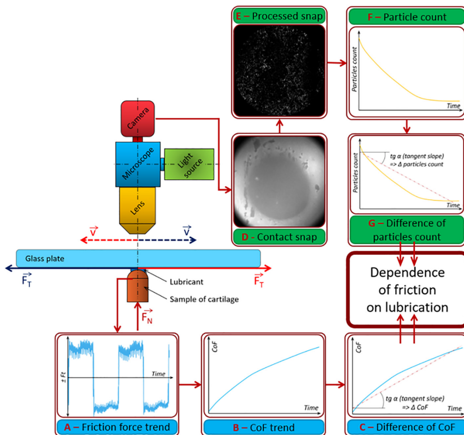
Fig. 4. Evaluation schema.
