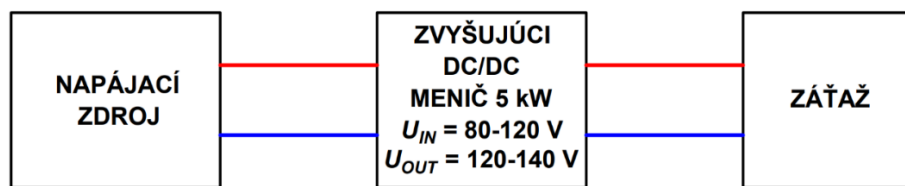
Obrázok 2.2 Blokova schéma s použitím zvyšujúceho meniča
