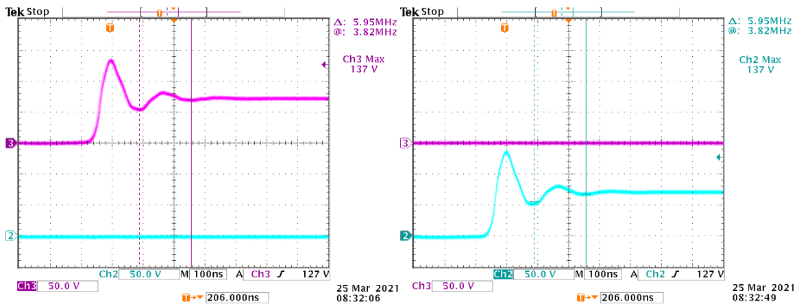
Obrázok 8.3 Detail priebehu napätia u_{DS} na tranzistoroch v synchronnom usmerňovači s RC snubbróm pri 60 W (vľavo TE, vpravo TF)
