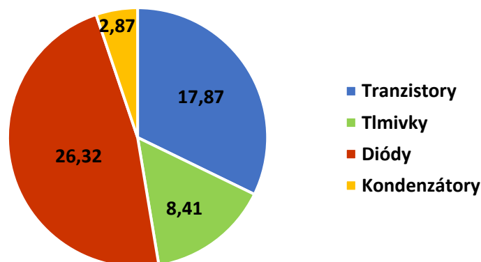
Celkové straty prekladaného zvyšujúceho meniča
