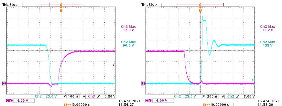
Obrázok 8.10 Detail priebehu napätí u_{GS} (CH3) a u_{DS} (CH2) na tranzistoroch TE pri výstupnom výkone 1 kW
