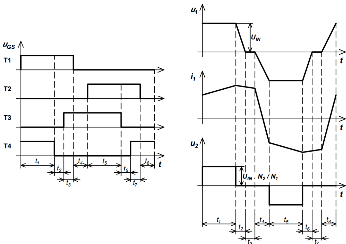
Obrázok 2.12 Priebiehy dvojjinného priepustného meniča – mäkké spínanie (prevzaté a upravené z [8])
