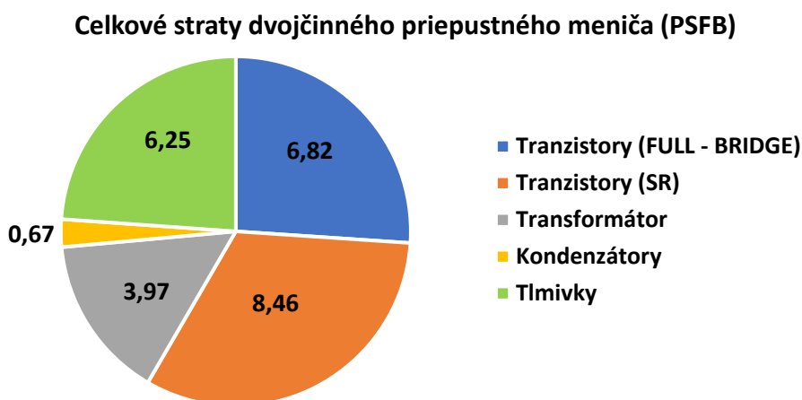
Obrázok 5.2 Grafický sumár strát dvojjinného priepustného meniča
