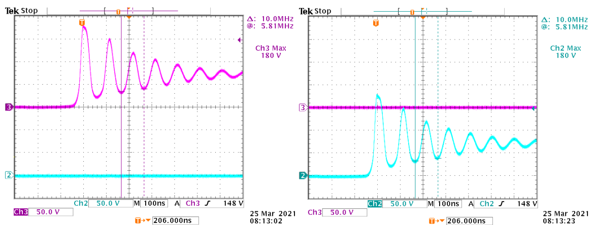
Obrázok 8.2 Detail priebehu napätia u_{DS} na tranzistoroch v synchronnom usmerňovači bez RC snubbru pri 60 W (vľavo TE, vpravo TF)
