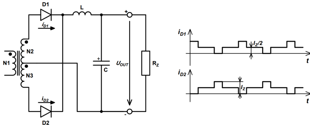
Obrázok 2.14 Dvojestný uzlový usmerňovač (prevzaté a upravené z [6])
