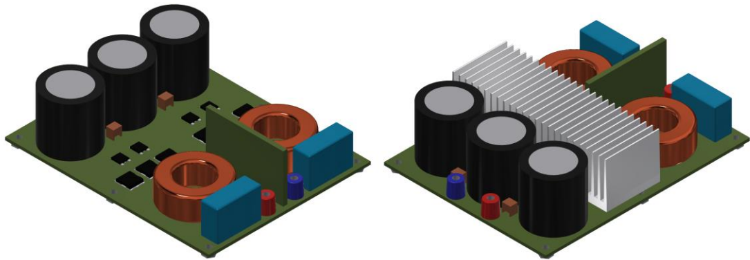
Obrázok 3.3 Prvotná vizualizácia prekladaného zvyšujúceho meniča
