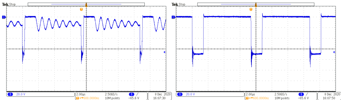
Obrázok 7.7 Priebehy napätí na sekundárnej usmerňovacej dióde v stave naprázdno (vľavo) a pri plnom odoberanom výkone (vpravo)
