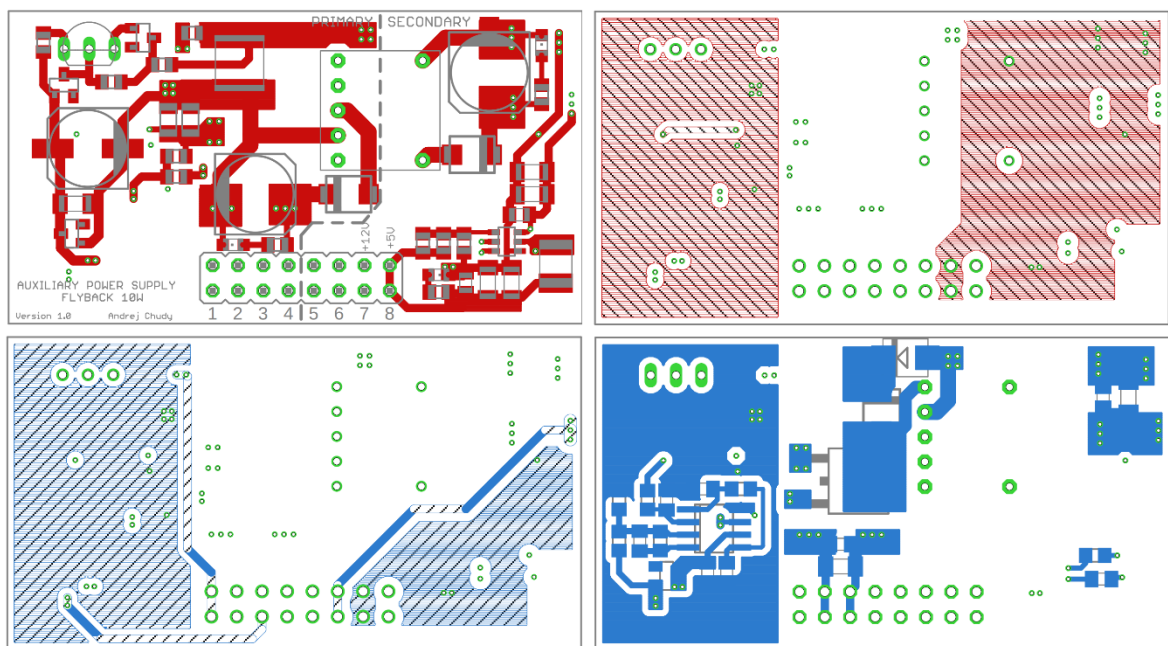
Obrázok 7.4 Jednotlivé vrstvy DPS pomocného zdroja
