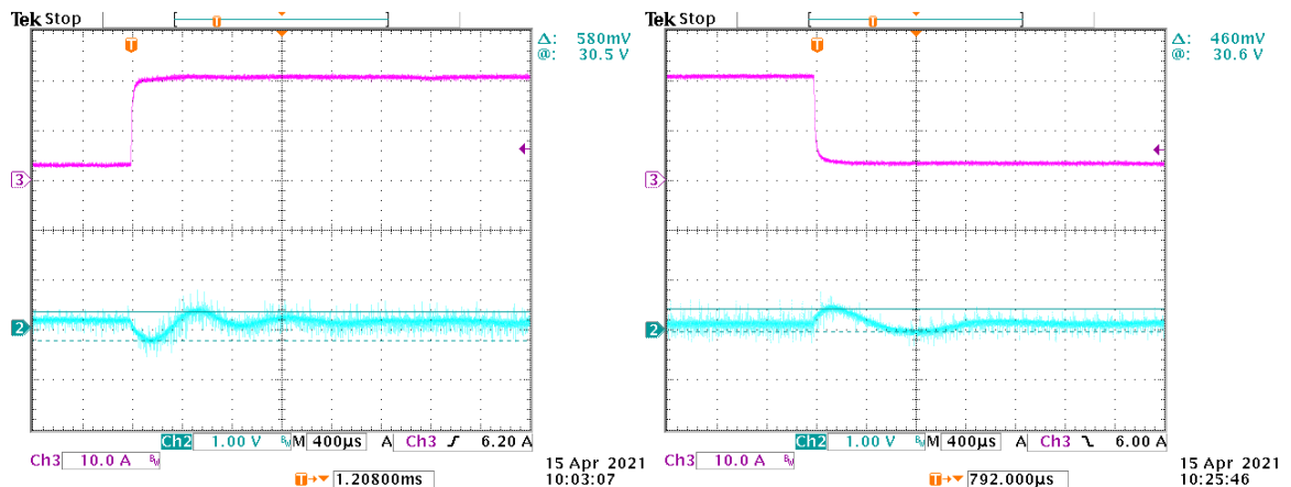
Obrázok 8.11 Skok záťaže z 10 % na 60 % (vľavo) a zo 60 % na 10 % menovitého prúdu/výkonu
