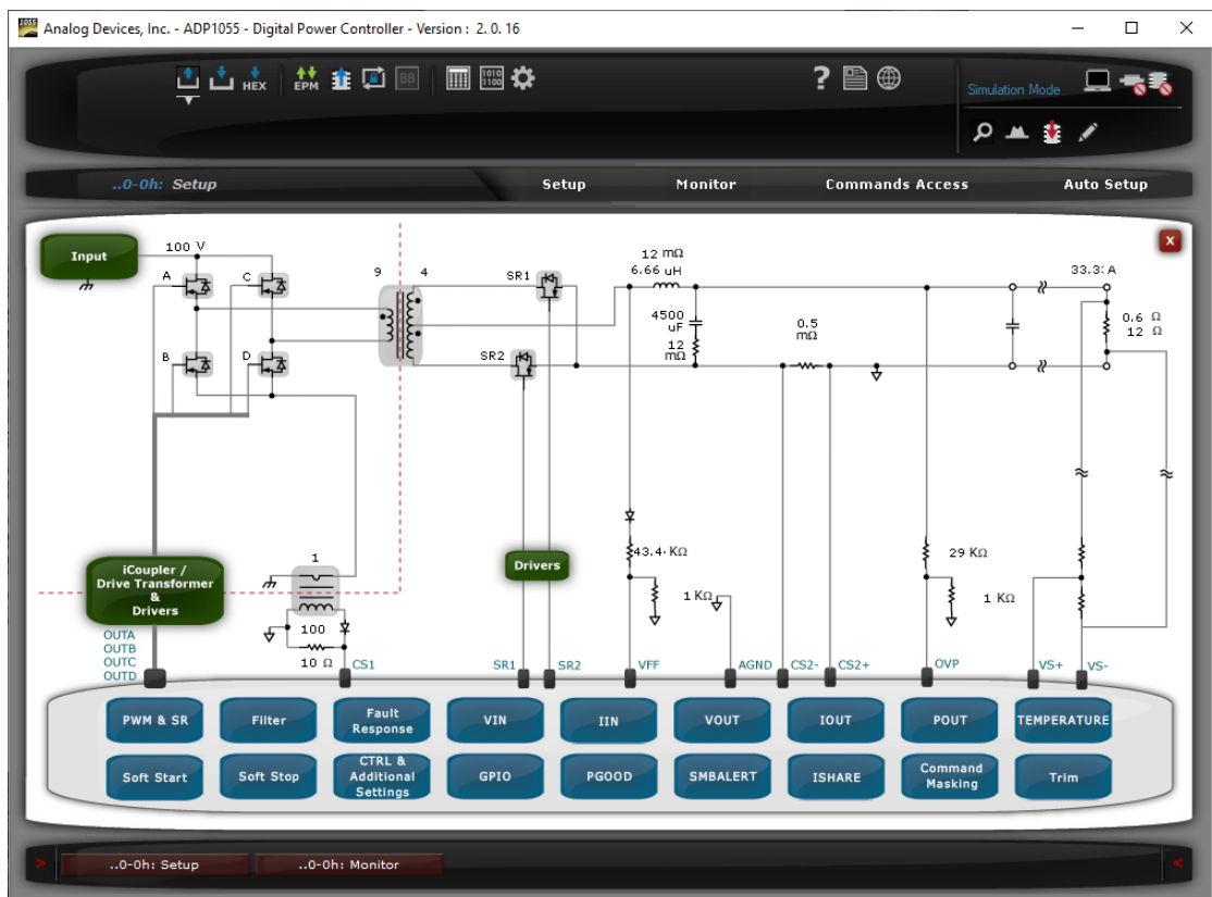
Obrázok 6.2 Grafické užívateľské rozhranie – GUI ADP1055
