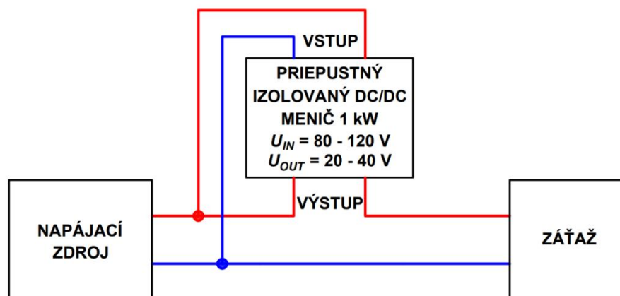
Obrázok 2.3 Blokova schéma s použitím priepustného izolovaného meniča
