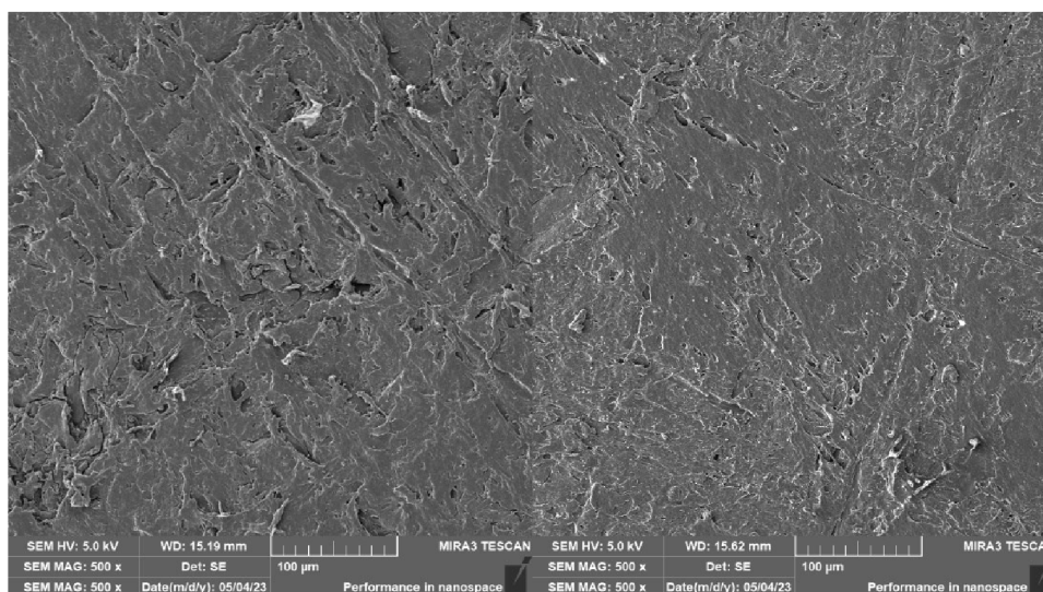
Obr. 4.13 Opotřebený povrch PHBV + 20 hm. % KN před (vlevo) a po stárnutí (vpravo)
