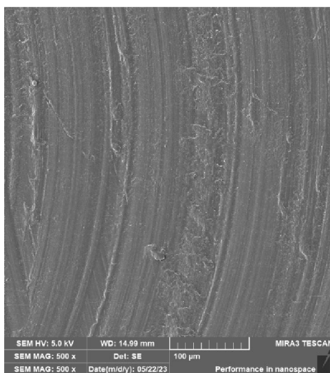
Obr. 4.14 Neopotřebený povrch PHBV po stárnutí
