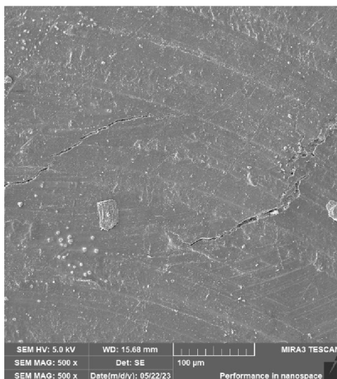
Obr. 4.12 Neopotřebený povrch PHBV + 20 hm. % RH po stárnutí
