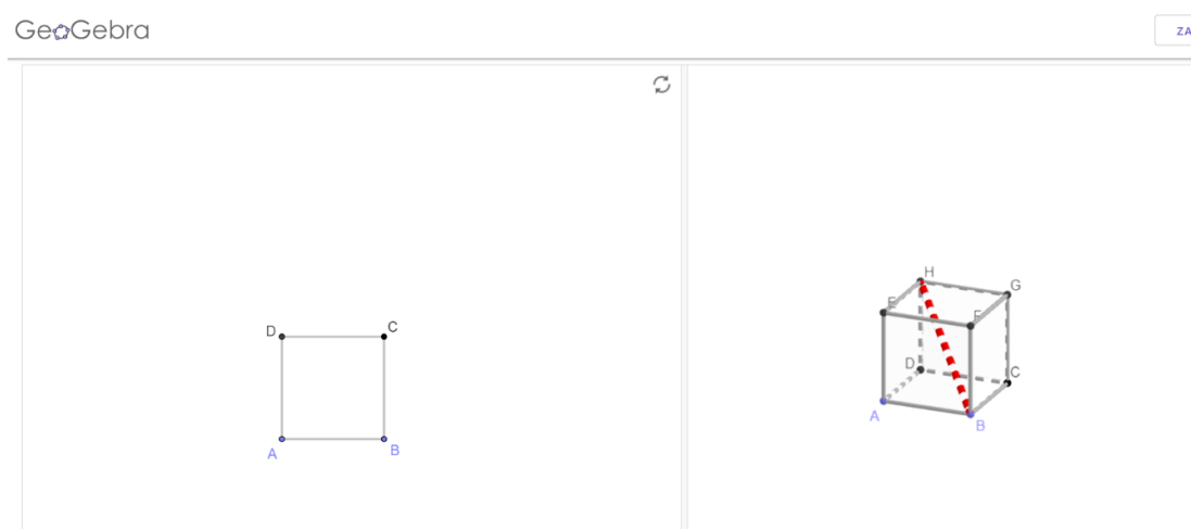
Obr. 21, znázornění Pythagorovy věty v Geogebře 1
