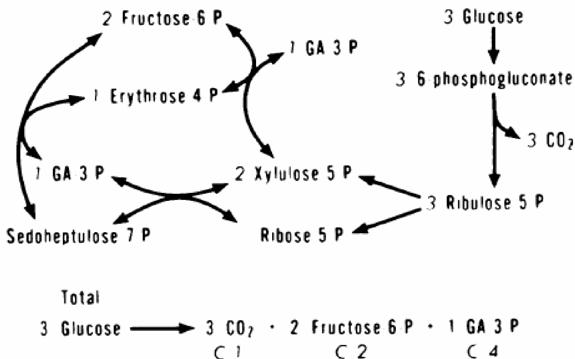
Obr. 3.4: Rovnováha uhlíka vychádzajúca z oxidácie troch molekúl glukózy cestou reakcií pentóзовého cykla A. tumefaciens [17]
