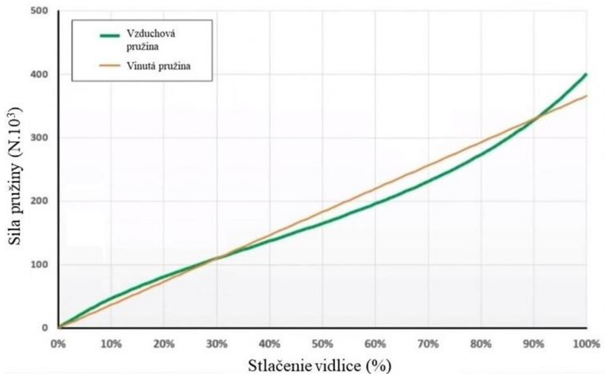
Obr. 2-2 Porovnanie priebehu pružnej sily vinutej pružiny so vzduchovou pružinou [5].
