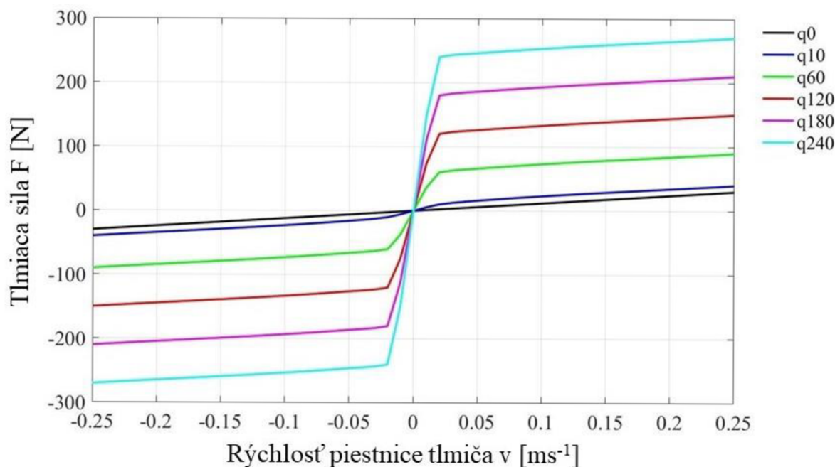
Obr. 5-7 Optimálne F-v charakteristiky MR tlmiča.
