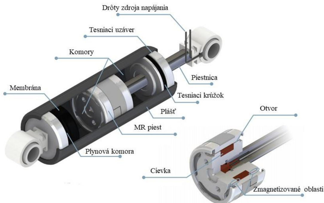
Obr. 2-9 Schematický model MR tlmica [22].
