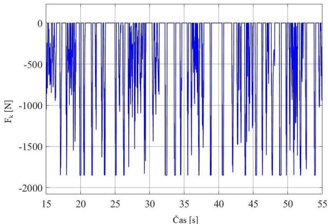
Obr. 5-5 Prítlačná sila zabezpečujúca trakciu kolesa.
