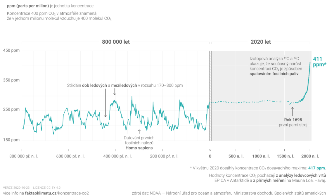
Obr. 1.5 Graf vývoje koncentrace CO 2 v atmosféře [14].
