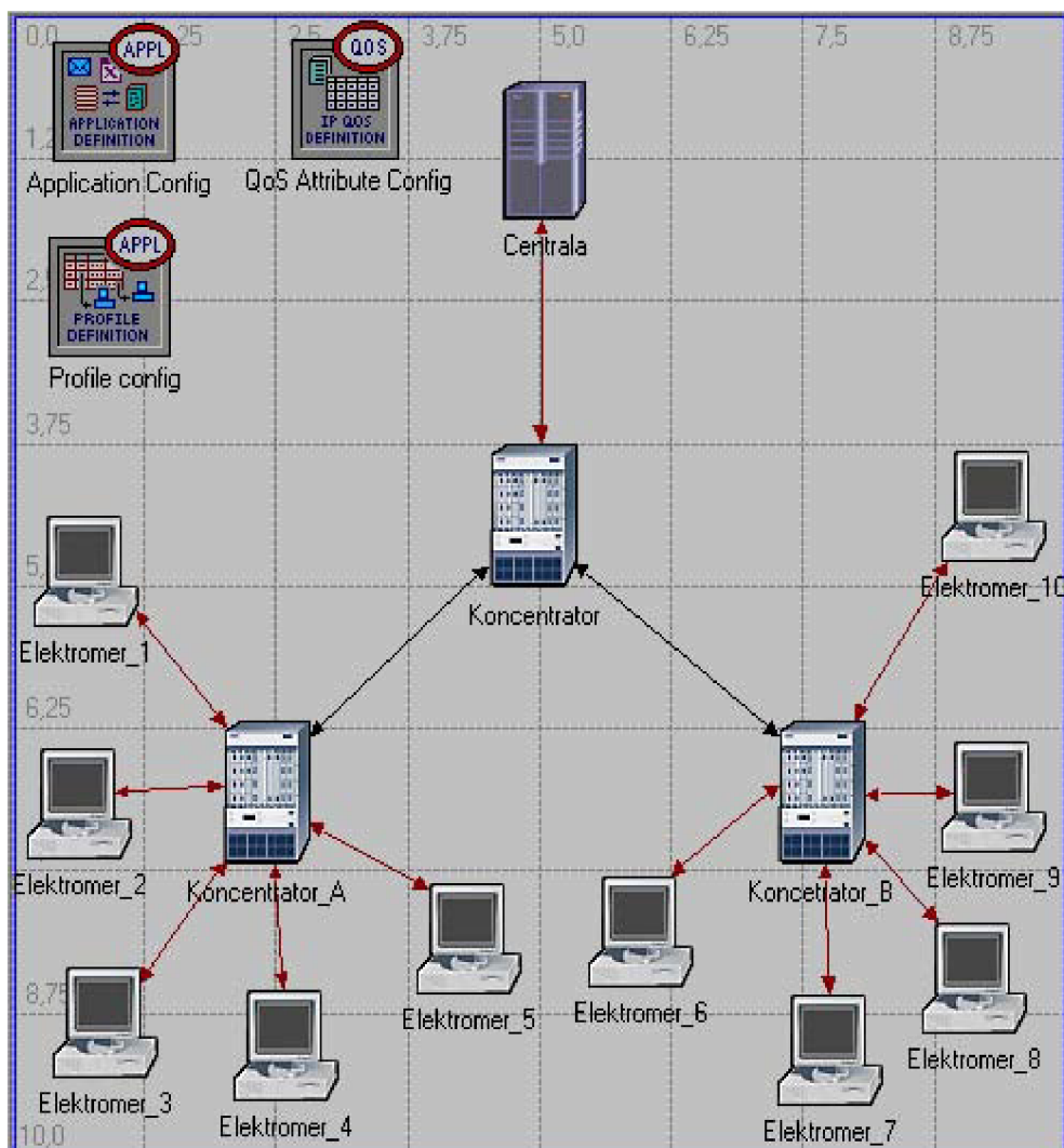
Obr. 5.1: Simulační síť
