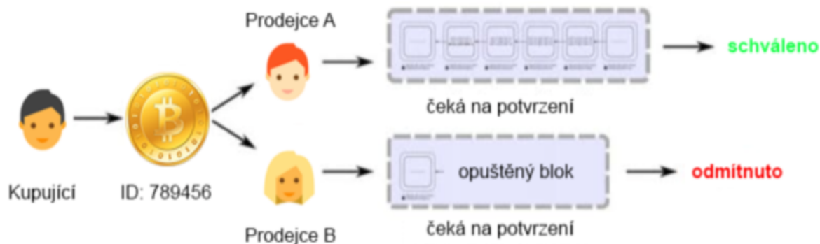
Obrázek 5: Schéma ochrany před dvojím utrácením (Zdroj: Finex.cz)
