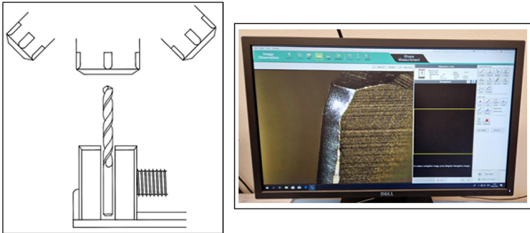
Obr.33 + 34 – Měření opotřebení vrtáku na mikroskopu + Vizualizace opotřebení
