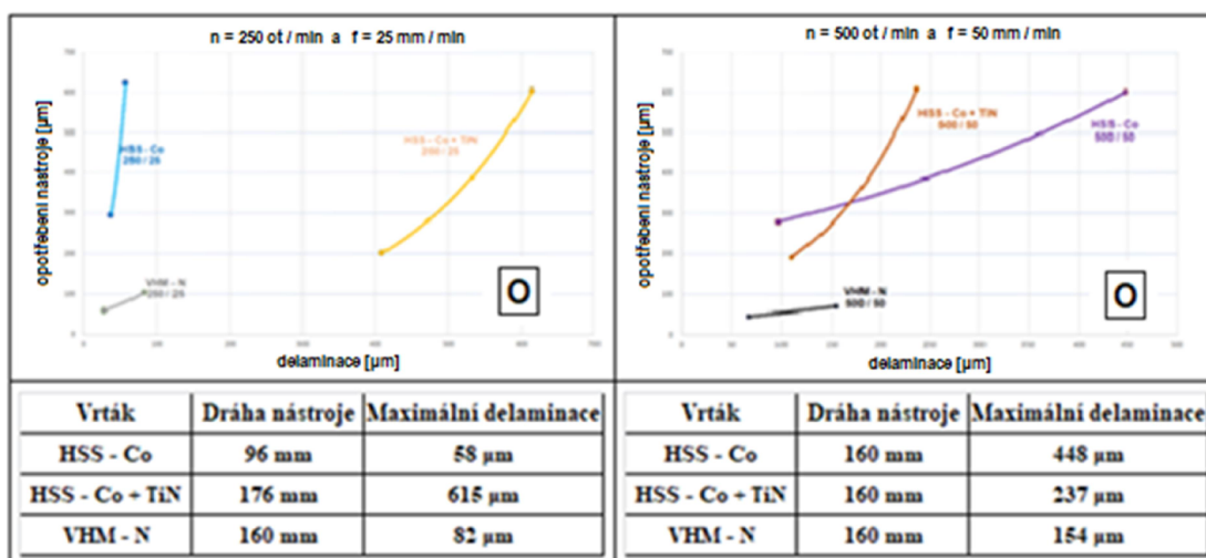
Obr.55 – Delaminace okrajů otvorů vzorků „O“ při „250/25“ a „500/50“
