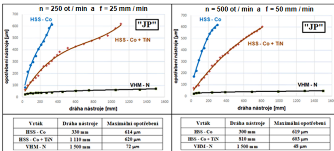
Obr.50 – Opatření nástrojů při obrábění vzorků „JP“ při „250/25“ a „500/50“
