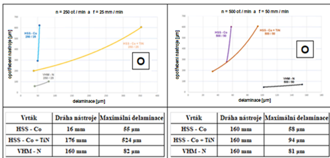
Obr.55 – Delaminace okrajů otvorů vzorků „O“ při „250/25“ a „500/50“
