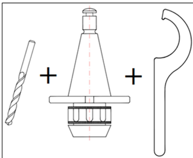
Obr.24 – Nástroj (vrták) + Sklíčidlo s kleštinou + Klíč
