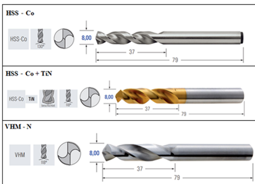
Obr.22 – Použité vrtáky
