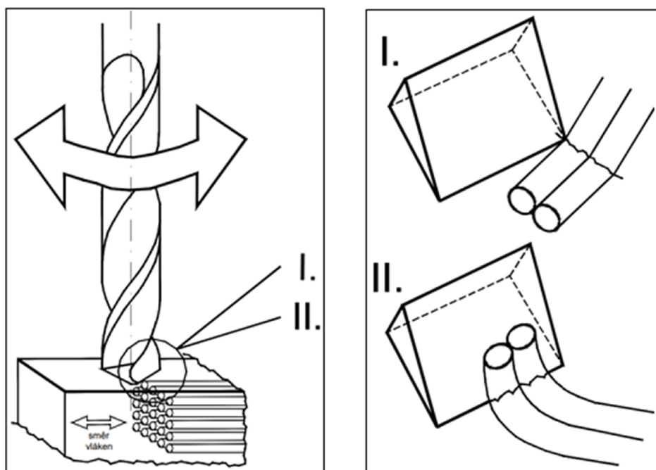
Obr.11 + 12 – Druhy opotřebení při vrtání – abraze a otěr [9]
