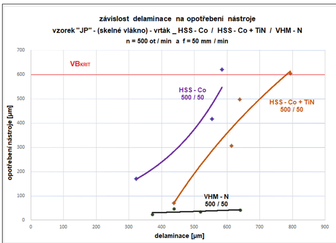
Graf.6 – Závislost delaminace okraje otvoru na opotřebení vrtáku HSS – Co / HSS – Co + TiN / VHM - N u vzorku „JP“ při „500/50“
