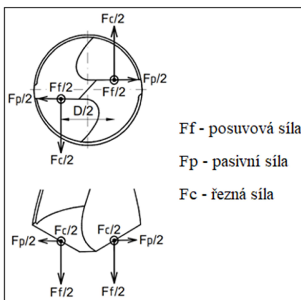
Obr.3 – Síly vznikající při vrtání u šroubového vrtáku [10]
