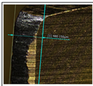
Obr.48 – Opotřebení na vrtácích HSS – Co + TiN
