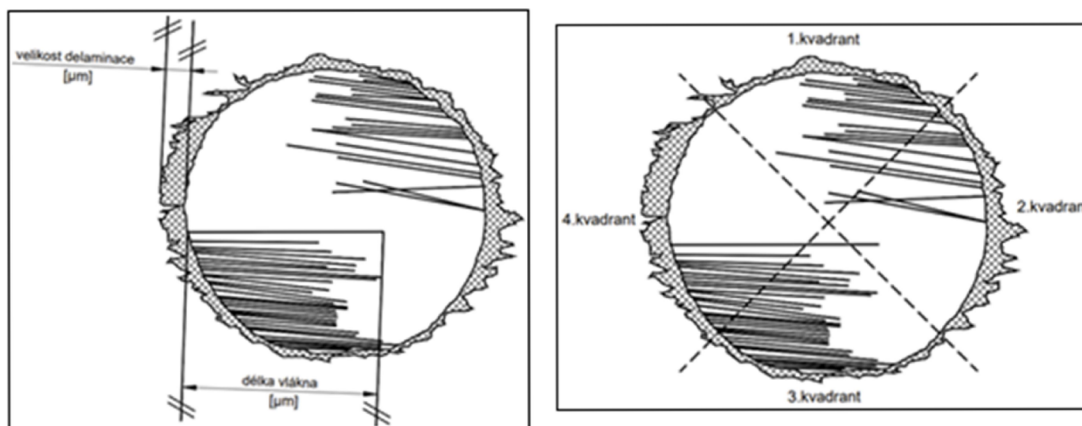
Obr. 37 + 38 – Měření delaminace – určení její velikosti a délek vláken výztuže vytažených z matrice a určení pozice
