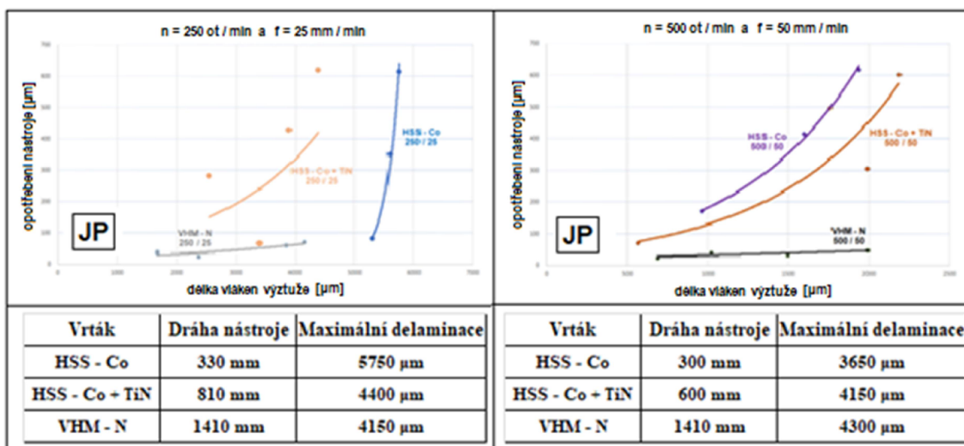
Obr.58 – Délky volných vláken výztuže u vzorků „JP“ při „250/25“ a „500/50“
