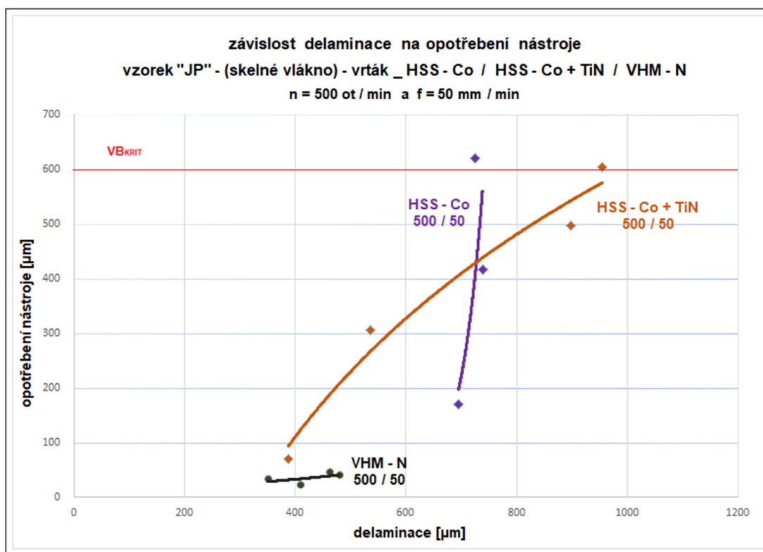
Graf.10 – Závislost delaminace okraje otvoru na opotřebení vrtáku HSS – Co / HSS – Co + TiN / VHM - N u vzorku „JP“ při „500/50“
