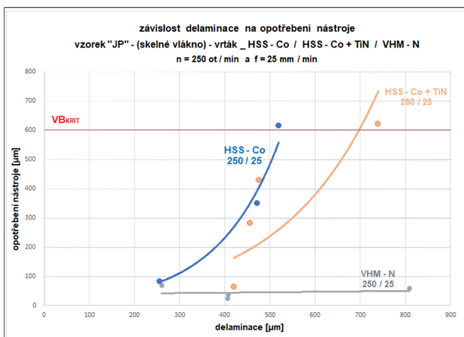
Graf.5 – Závislost delaminace okraje otvoru na opotřebení vrtáku HSS – Co / HSS – Co + TiN / VHM - N u vzorku „JP“ při „250/25“
