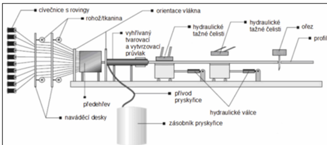
Obr.6 – Linka pro výrobu materiálu pultruzí [14]
