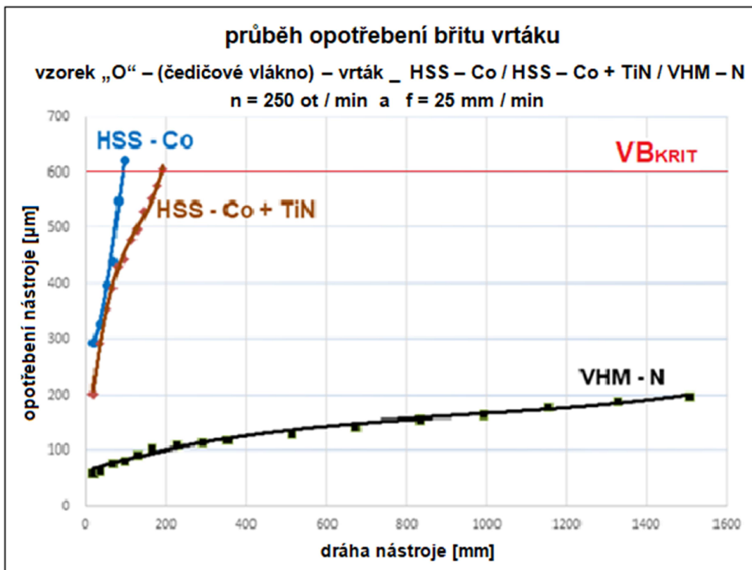
Graf.2 – Opotřebení na vrtáku HSS – Co / HSS – Co + TiN / VHM - N u vzorku „O“ při „250/25“
