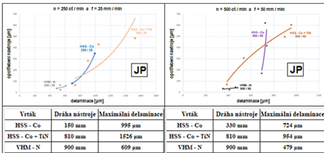
Obr.54 – Delaminace okrajů otvorů vzorků „JP“ při „250/25“ a „500/50“
