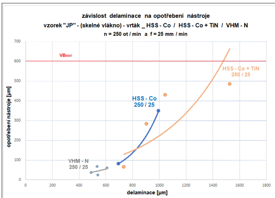
Graf.9 – Závislost delaminace okraje otvoru na opotřebení vrtáku HSS – Co / HSS – Co + TiN / VHM - N u vzorku „JP“ při „250/25“
