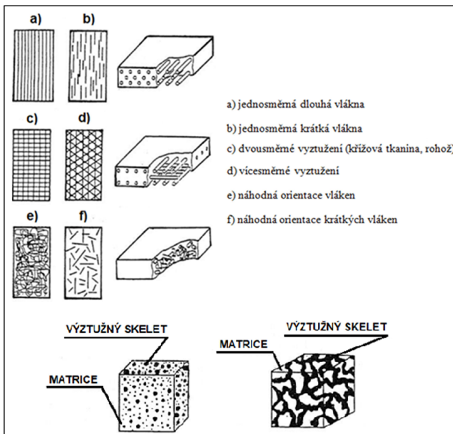
Obr. 4 – Typy vláknových vyztuží, částicový a skeletový kompozitní materiál [15]
