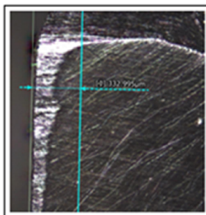
Obr.47 – Opotřebení na vrtácích HSS – Co
