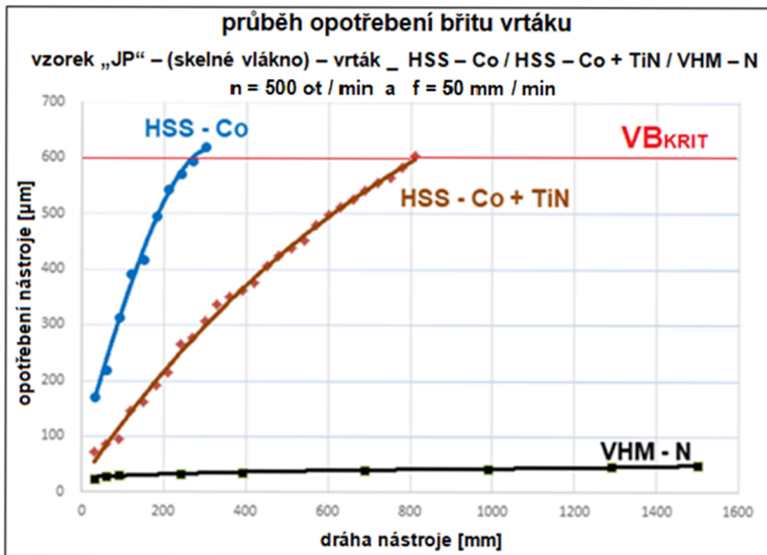
Graf.3 – Opotřebení na vrtáku HSS – Co / HSS – Co + TiN / VHM - N u vzorku „JP“ při „500/50“
