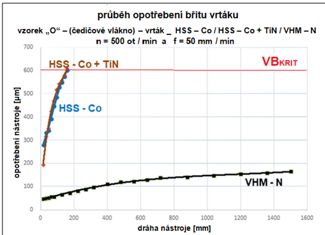
Graf.4 – Opatření na vrtáku HSS – Co / HSS – Co + TiN / VHM - N u vzorku „O“ při „500/50“
