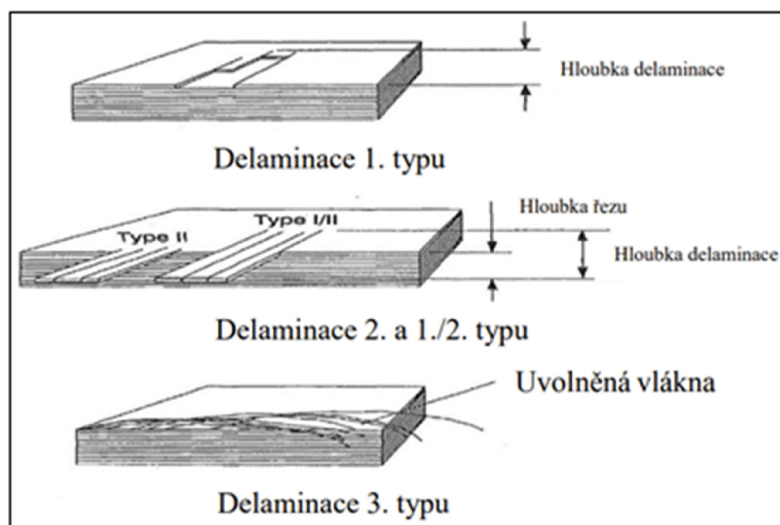
Obr.7 – Typy delaminace [17]
