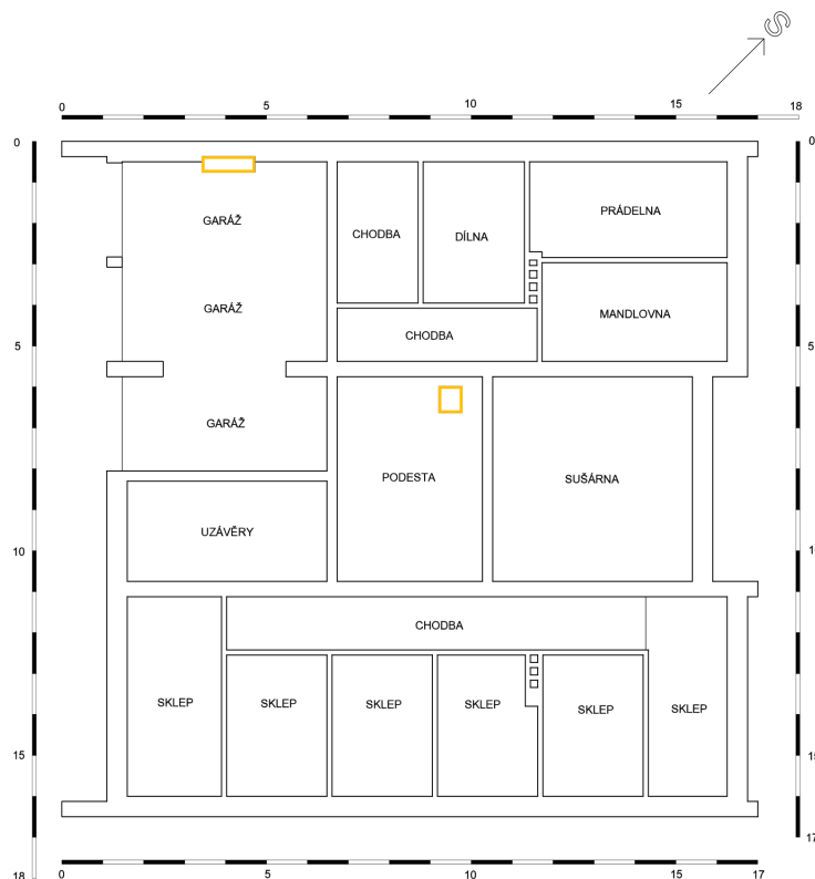
Obr. 3.4: Pôdorys suterénu
