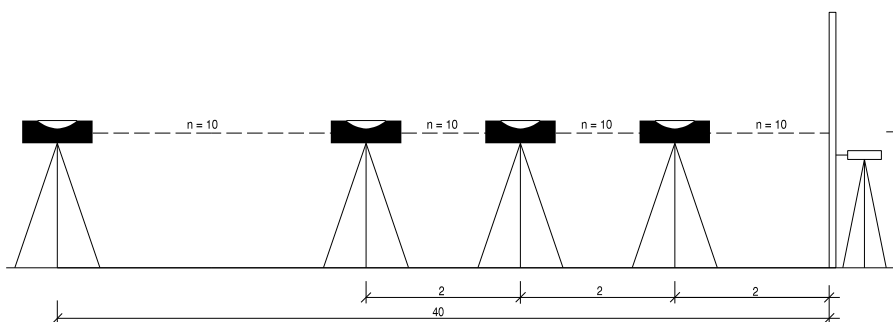
Obr. 3.17: Schéma experimentu vplyvu dĺžky zámery na presnosť čítania na stupnici
