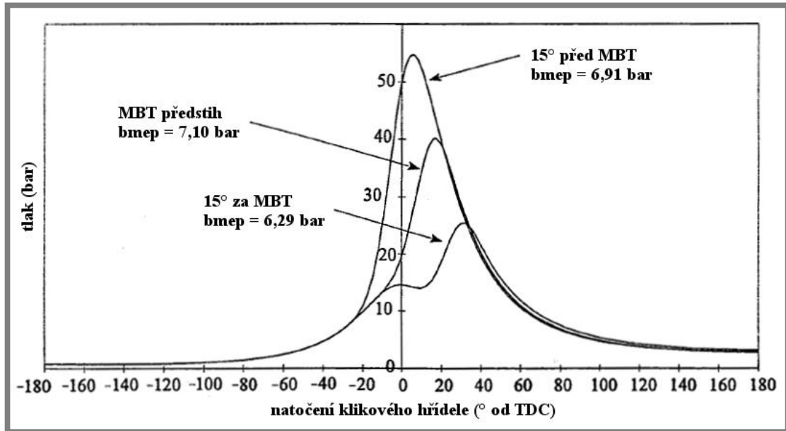
Obr. 7 Předčasný a pozdní předstih v porovnání s MBT hodnotou v p-α diagramu [1]
