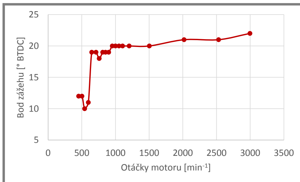
Graf 1 Naměřená charakteristika předstihu
