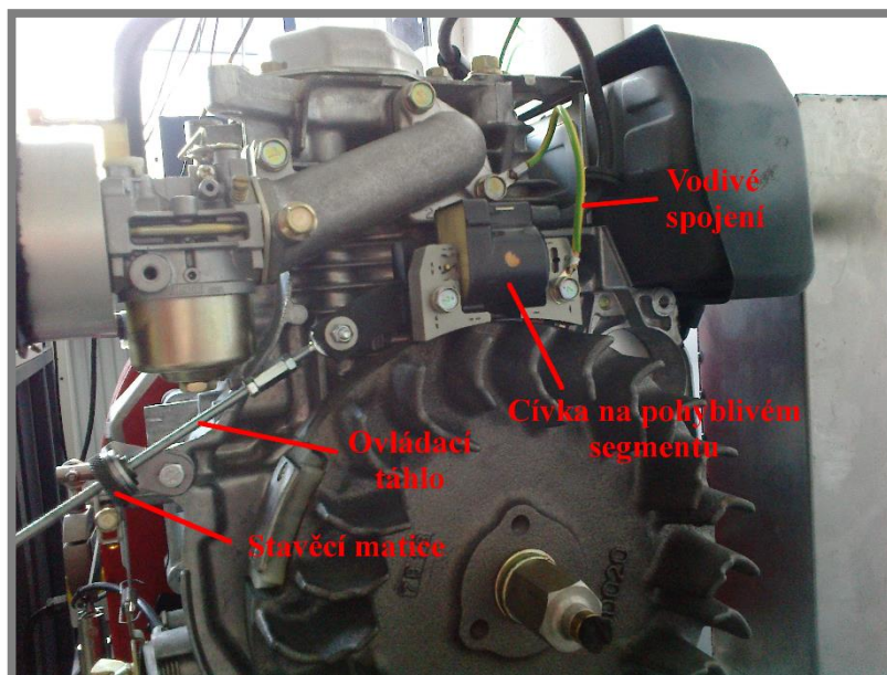
Obr. 21 Zkompletovaný mechanismus
