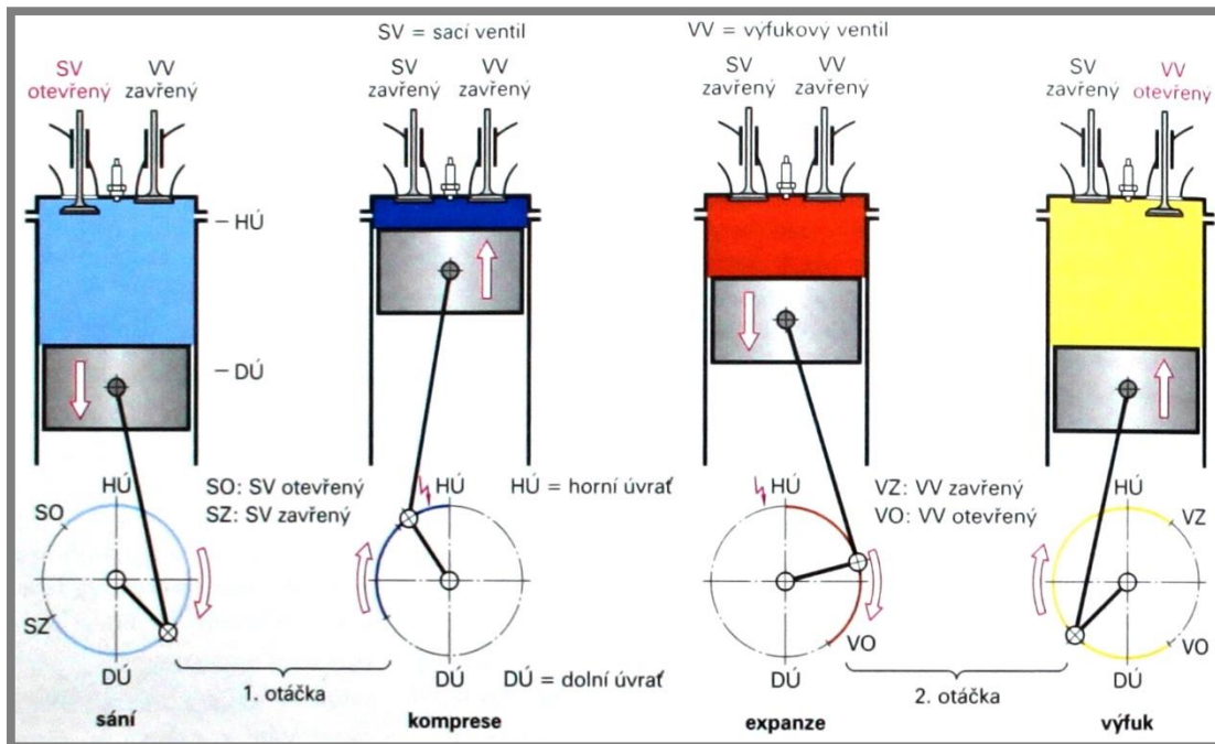
Obr. 1 Pracovní cyklus čtyřtakového motoru [2]
