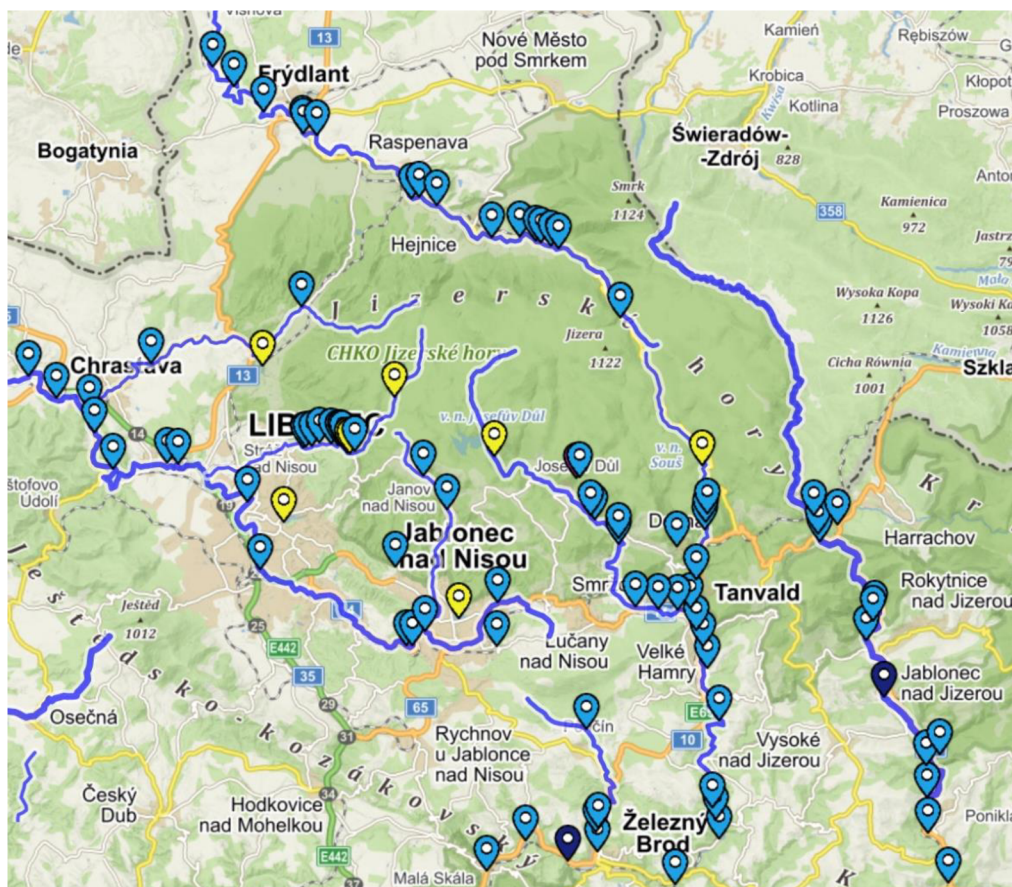
Obr. 12 Situační mapa MVE v oblasti Jizerských hor a Liberecka [8]
