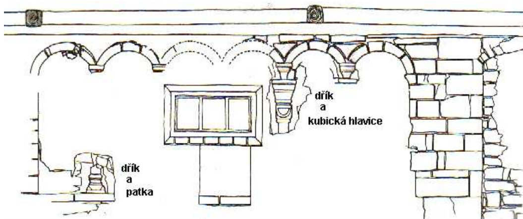
Obr. 10 Postoloprty, farní stodola, situační kresba šestiobloukového románského okna s hlavicemi, sloupky a patkami (Převzato Římskokatolická farnost – děkanství Postoloprty a farnost Lenešice. URL: http://postoloprty.farnost.cz/kostely-a-kaple/kostel-nanebevzeti-panny-marie/ )
