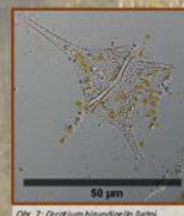
Obr. 7: Gracilaria minutula (letní plankton rybníka Staně Bahno)
