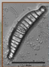
Obr. 12: Epithemia oshata (jarní nárost na hrázi - rybník U Mlýna)
