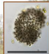
Obr. 4: Microcystis sp. (letní plankton středního rybníka Na Bubně)
