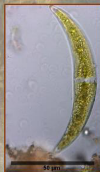
Obr. 11: Closterium moniliferum (jarní plankton rybníka U Mlýna)
