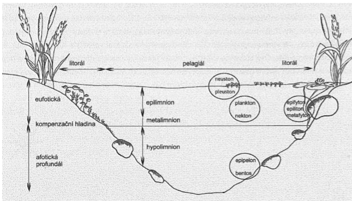
Obr. 4 Letní stratifikace dimiktické nádrže (Pouličková 2011)
