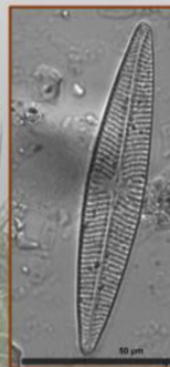
Obr. 14: Nitzschia radiosa (podzimní nárost na mlči - rybník U Mlýna)
