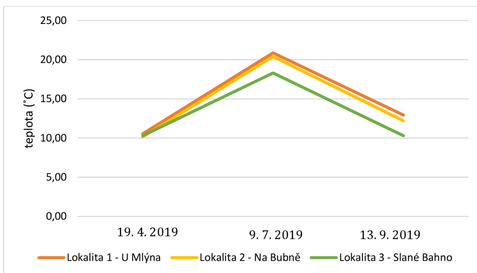
Graf 1 Porovnání naměřených hodnot teplot na jednotlivých lokalitách U Mlýna, Na Bubně a Slané Bahno během třech odběrů v roce 2019 (vlastní tvorba).
