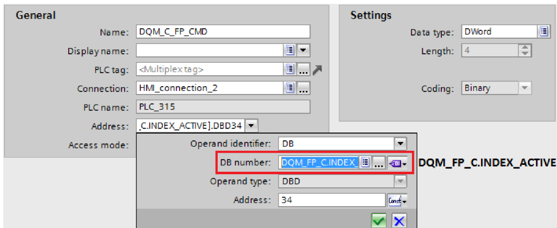
Obr. 6.4) Znáoznenie princípu adresového multiplexovania tagu DQM_FP_CMD
