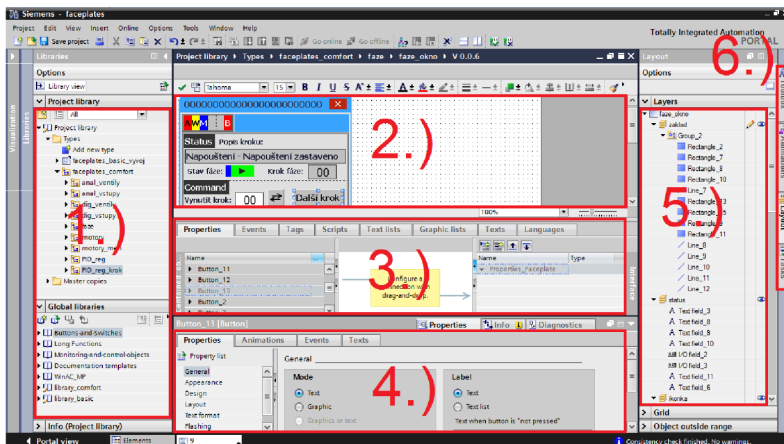
Obr. 5.1) Pracovné okno pre tvorbu faceplate
