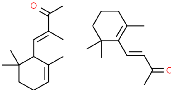
Obrázek 11: alfa-jonon [36]
