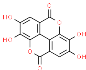
Obrázek 6: Struktura kyseliny ellagové [23]
