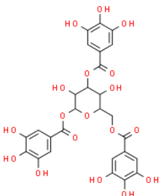
Obrázek 10: Struktura 1,3,6 – Tris-O-(3,4,5-trihydroxybenzoyl)hexopyranosy (př. gallotaninu) [31]
