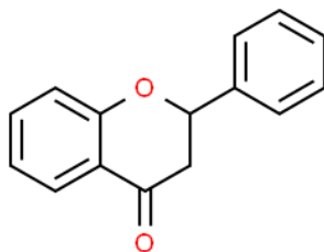
Obrázek 5: Struktura flavanonu [21]
