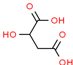
Obrázek 2: Struktura kyseliny jablečné [14]
