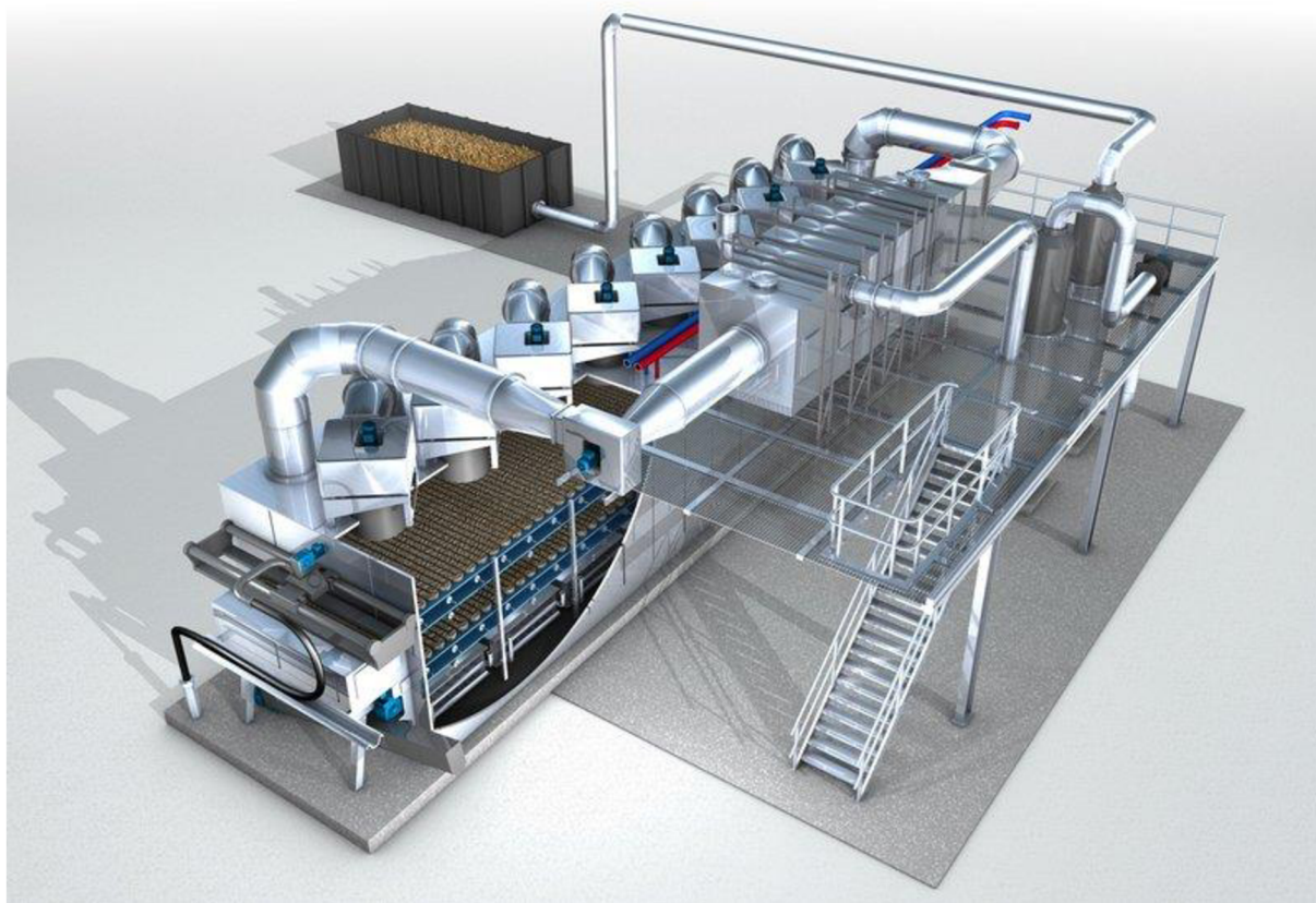
Obrázek 5: Nizkoteplotní pásová sušárna (zdroj: [31])
