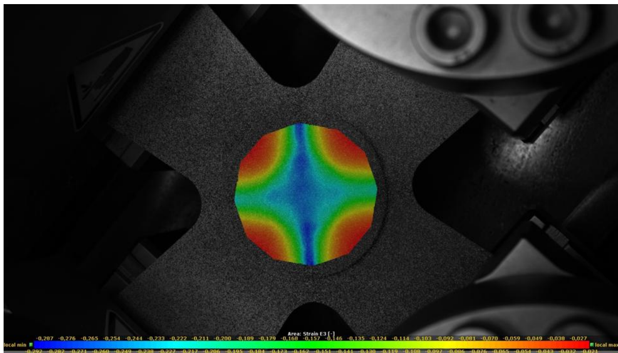
Obr. 3.17 Znáznornění deformací v průběhu zkoušky v programu MercuryRT.
