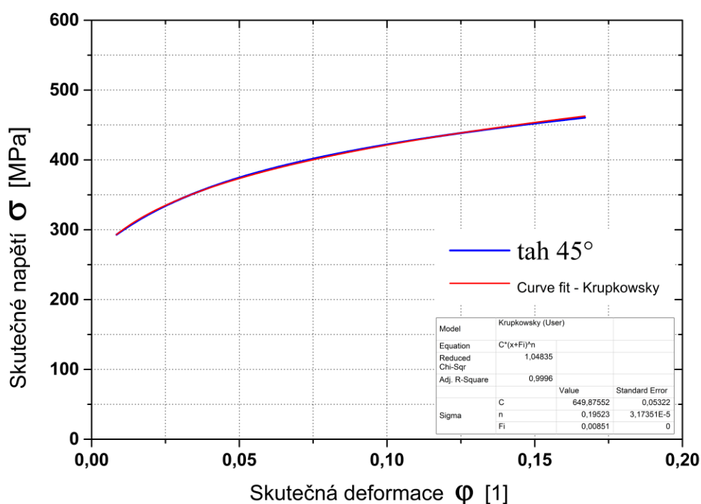
Obr. 3.3 Příklad použití matematické funkce Swift-Krupowski pro stanovení aproximační křivky a zjištění koeficientu monotónního zpevnění, exponentu deformačního zpevnění a ofsetové deformace, konkrétně pro vzorek ze směru 45°. V tabulce jsou uvedené deformační hodnoty.
