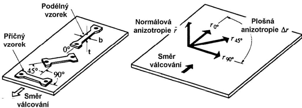
Obr. 2.12 Znáznornění odběru vzorků pro zkoumání anizotropie [17]
