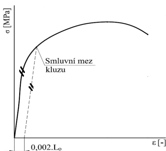
Obr. 2.2 Určování smluvní meze kluzu v diagramu []
