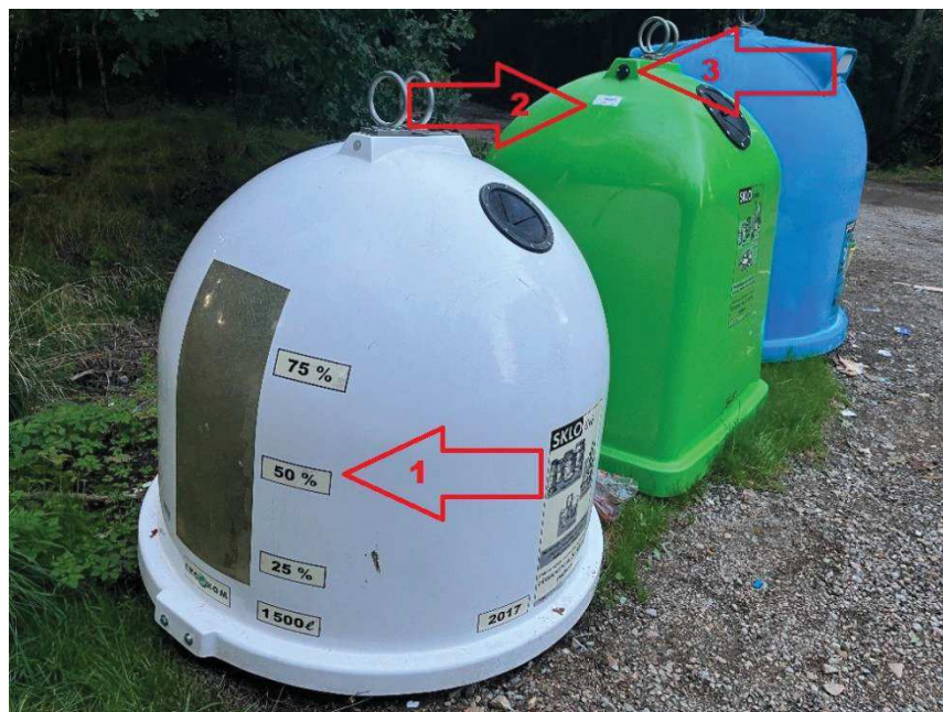
Obrázek 18 - Kontejnery ve městě Rokycany, šipka č.1: stupnice zaplněnosti, šipka č.2: čárový kód s identifikačními údaji kontejneru, šipka č.3: RFID čip
