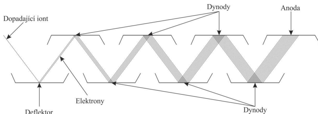
Obr. 3 Schéma elektronásobiče s oddělenými dynodami [3]
