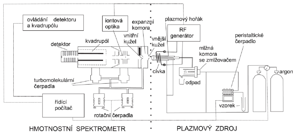
Obr. 1 Schéma ICP-MS [3]
