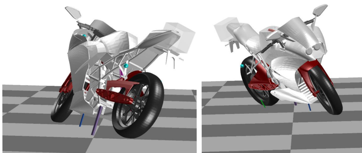
Obr. 2.3 3D zobrazení inverzního modelu motocyklu, průjezd zatáčkou
