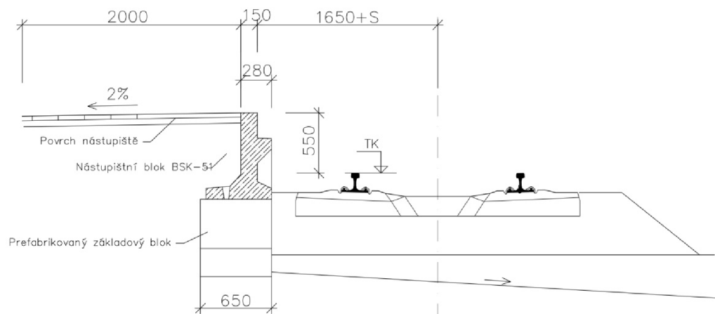
Obr. č. 15: Nástupištní blok BSK – 51
