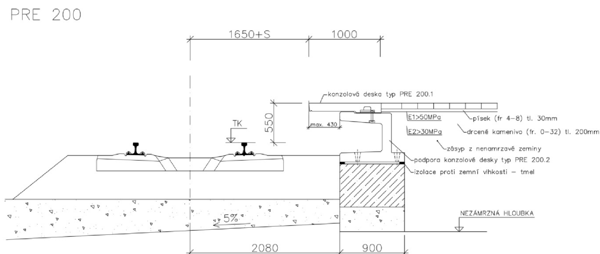
Obr. č. 11: Nástupiště PRE 200
