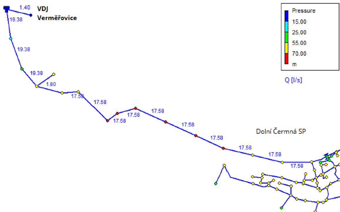
Obr. 4.16 Hydraulické poměry: VDJ Verměřovice – Dolní Čermná, nové čerpadlo
