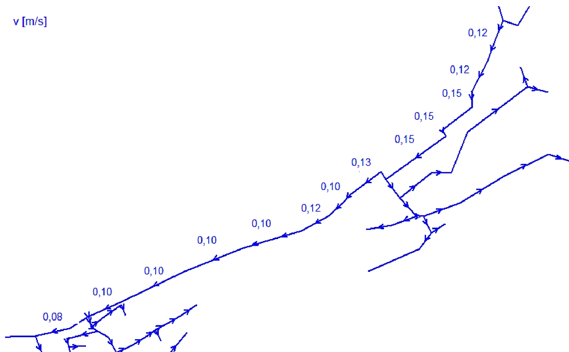
Obr. 4.19 Rychlost proudění vody v potrubí: Dolní Čermná – stávající stav
