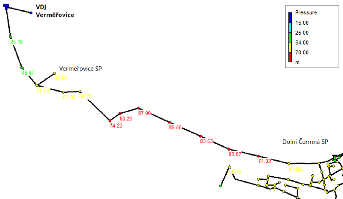
Obr. 4.9 Hydraulická analýza: tlakové poměry VDJ Verměřovice - Dolní Čermná
