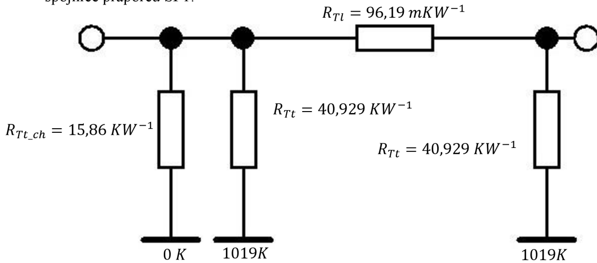
Obrázek 4.4 Kompletní tepelné schéma SP1
