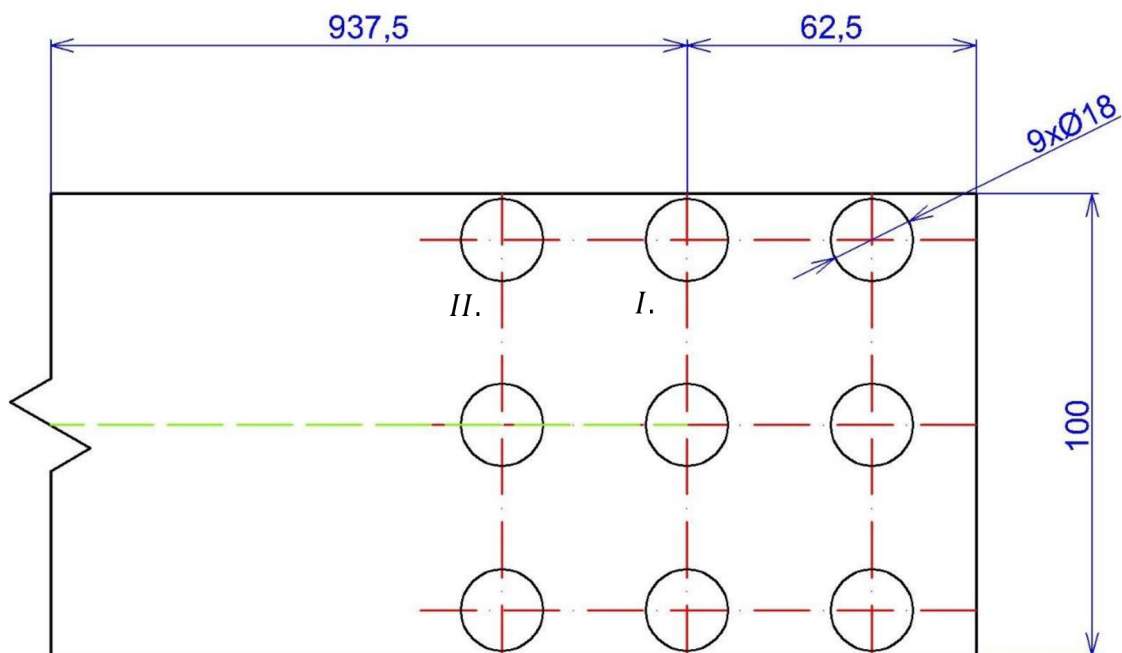
Obrázek 4.1 Přívodní pásovina
