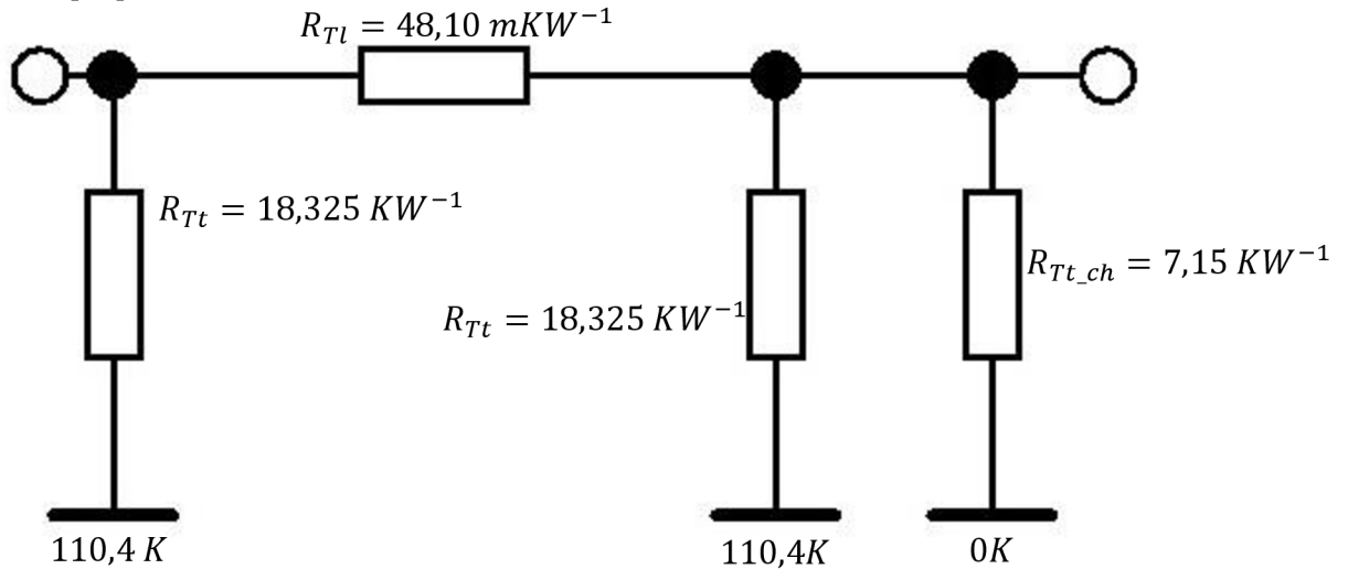
Obrázek 4.5 Kompletní tepelné schéma SP2
