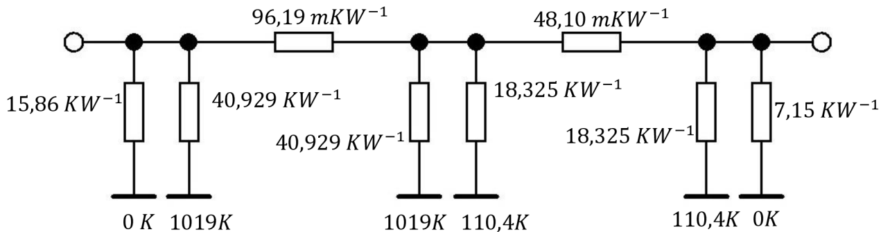
Obrázek 4.6 Kompletní tepelné schéma přívodní svorky
