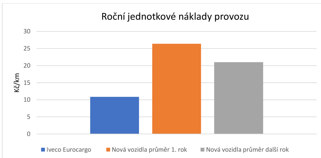
Obrázek 21 – Graf porovnání jednotkových ročních nákladů vozidel
