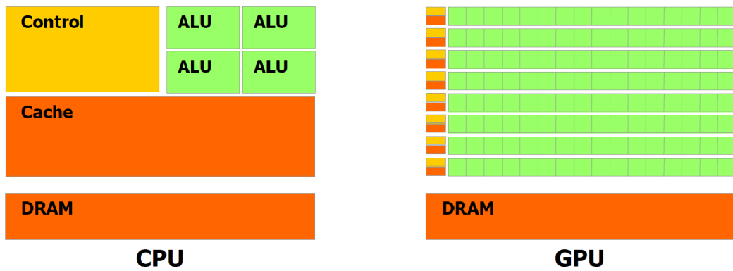
Obrázok 2.2: Rozdielna štruktúra GPU a CPU (prevzaté z [2])
