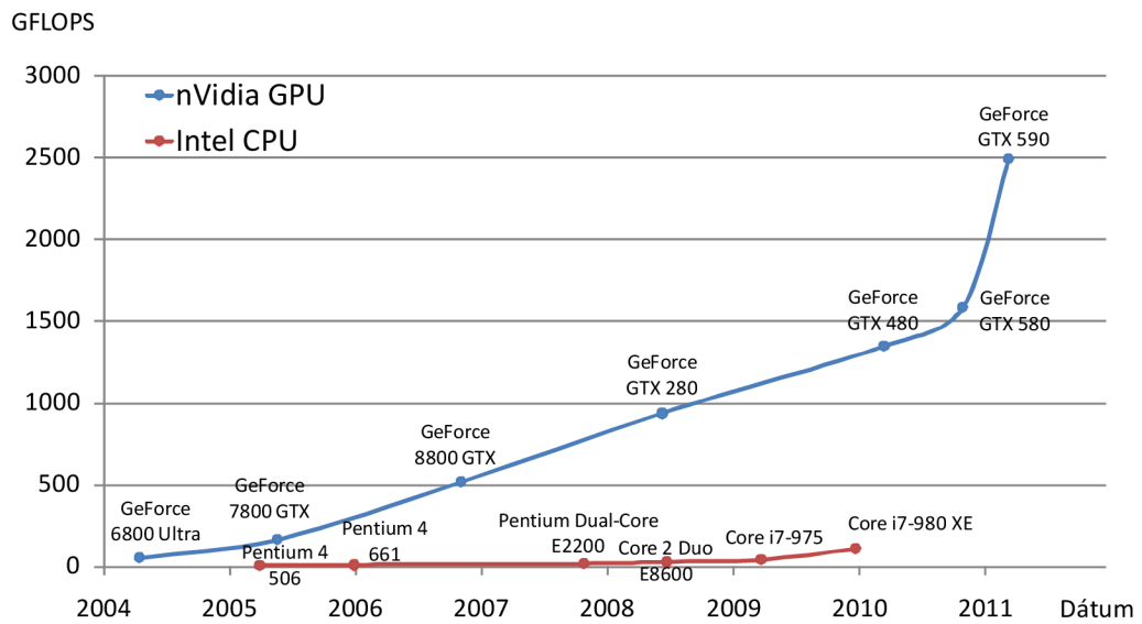
Obrázok 2.1: Porovnanie rozdielu výkonu GPU a CPU pri práci s číslami v pohyblivej rádovej čiark
