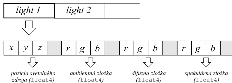
Obrázok 6.1: Štruktúra uloženia svetelných zdrojov na GPU
