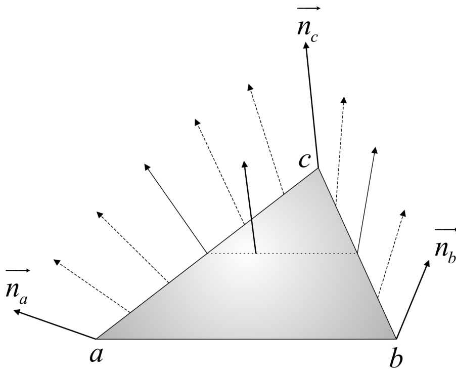
Obrázok 3.9: Phongovo tieňovanie
