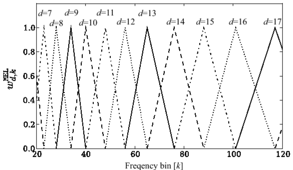
Obrázok 1: Nenormalizovaná banka filtrov [2].
