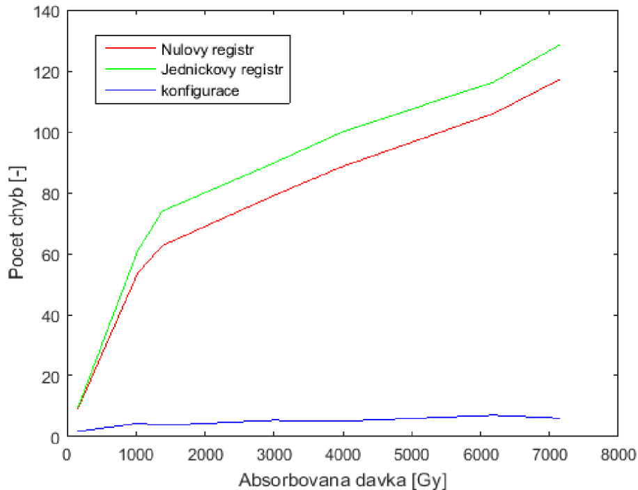
Obr. 31: Vývoj počtu chyb – střední hodnota
