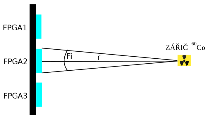
Obr. 27: Náčrt ozařovacího pracoviště
