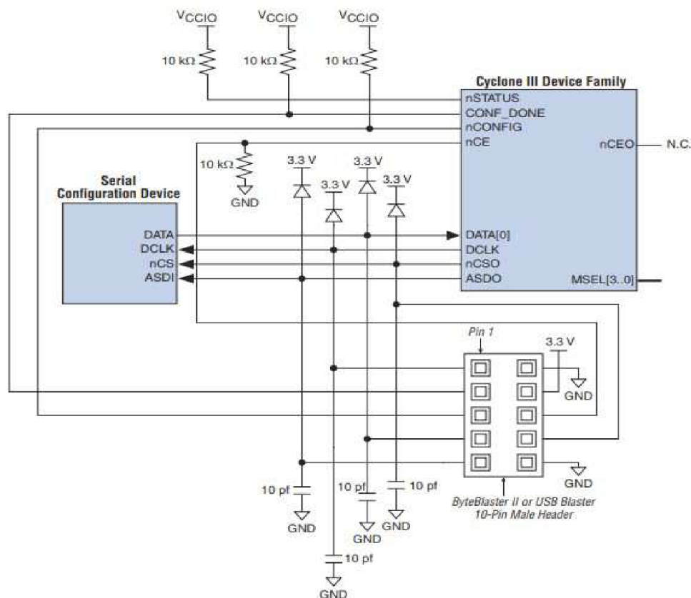
Obr. 20: In system programování konfigurační flash paměti [16]
