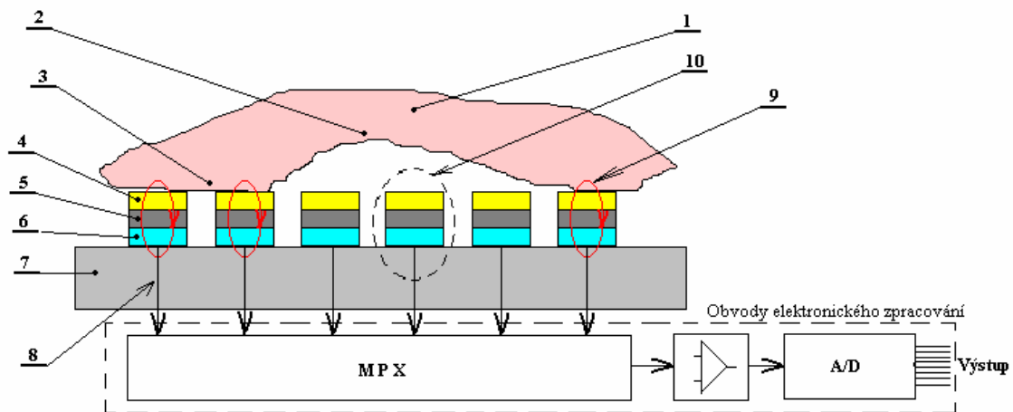
Obr. 12: Obrázek zachycující činnost odporového snímače otisku prstu.
