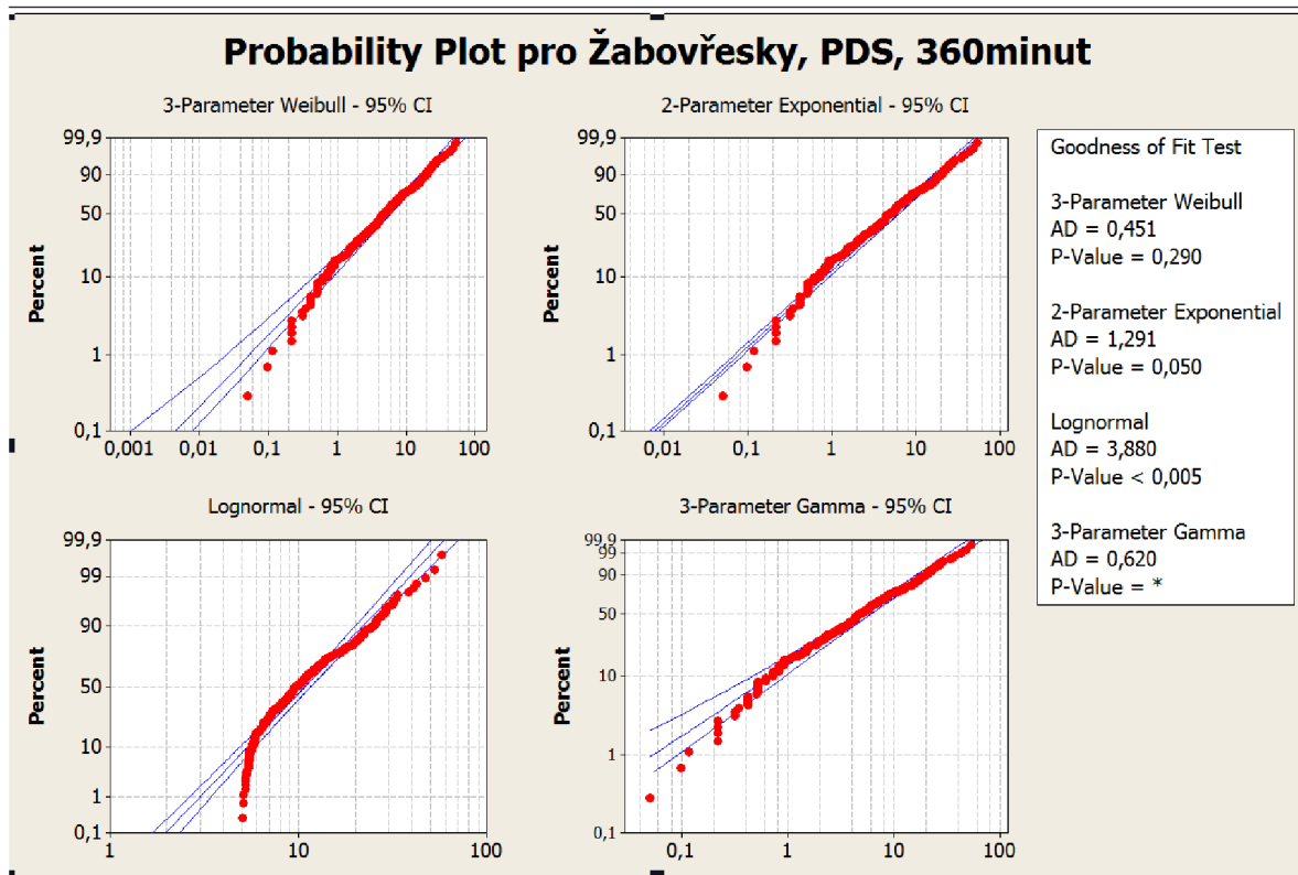
Obrázek 6.4: Některé probability plots pro 360 minutovou dešťovou řadu ze stanice Brno - Žabovřesky. Řada obsahuje pouze hodnoty vyšší než 5.
