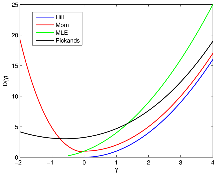
Obrázek 5.8: Asymptotický rozptyl.
