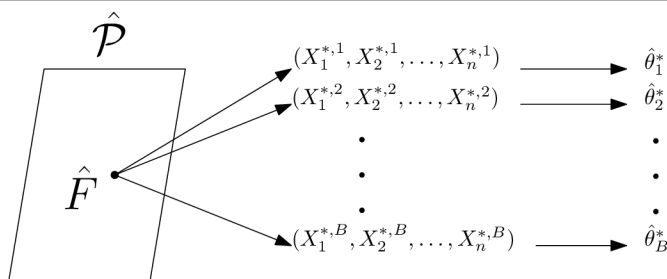
Obrázek 4.2: Schéma bootstrap
