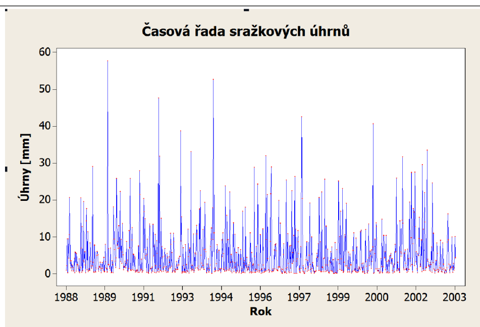
Obrázek 6.1: Časová řada 16ti let vyvzorkovaných srážkových úhrnů trvajících 360 minut ze stanice Brno - Žabovřesky. Celkem 781 měření.
