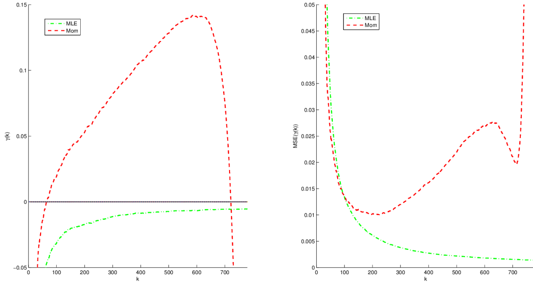
Obrázek 6.8: Simulace z exponenciálního rozdělení o rozsahu 781 s počtem opakování R = 5 krát MC = 500 . Průměrné odhady parametru \gamma v závislosti na k (vlevo). Střední kvadratická chyba v závislosti na k (vpravo).
