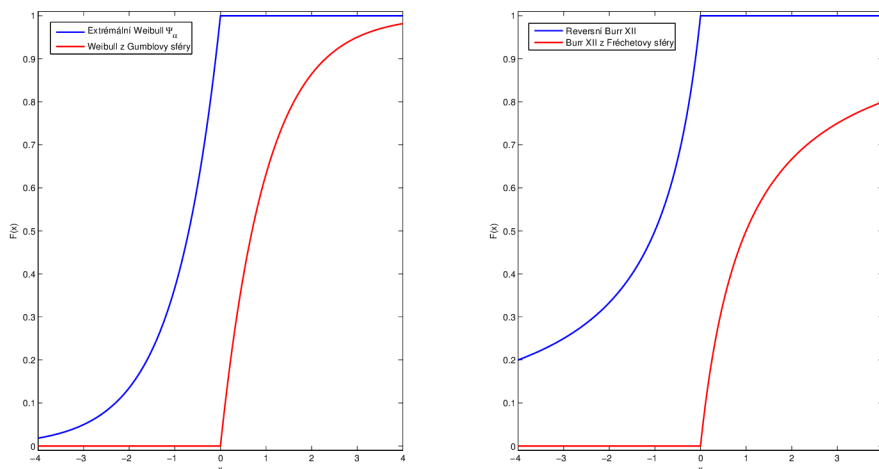
Obrázek 3.6: Srovnání distribučních funkcí. Vlevo extrémální ( \gamma = -1 ) a obyčejné ( \gamma = 0 ) Weibullovo rozdělení; \alpha = 1 . Vpravo reversní ( \gamma = -1 ) a obyčejné ( \gamma = 1 ) Burrovo rozdělení typu XII; \lambda = \tau = 1 .
