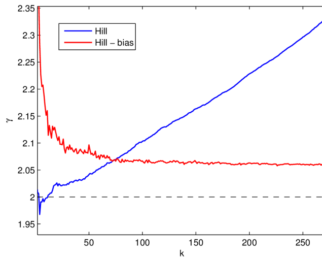
Obrázek 5.6: Průměrný Hillův odhad a průměrný opravený Hillův odhad \overline{\hat{\gamma}_H^C} na simulovaných datech rozsahu n = 1000 z rozdělení \text{Burr}(1, -\rho, \frac{1}{-\rho\gamma}) (typ XII) s parametrem tvaru \gamma = 2 a \rho = -0.5 .
