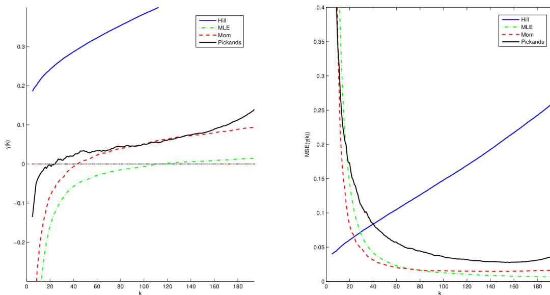
Obrázek 6.5: Simulace z Weibullova rozdělení o rozsahu 781 s počtem opakování R = 5 krát MC = 500 . Průměrné odhady parametru \gamma v závislosti na k (vlevo). Střední kvadratická chyba v závislosti na k (vpravo).
