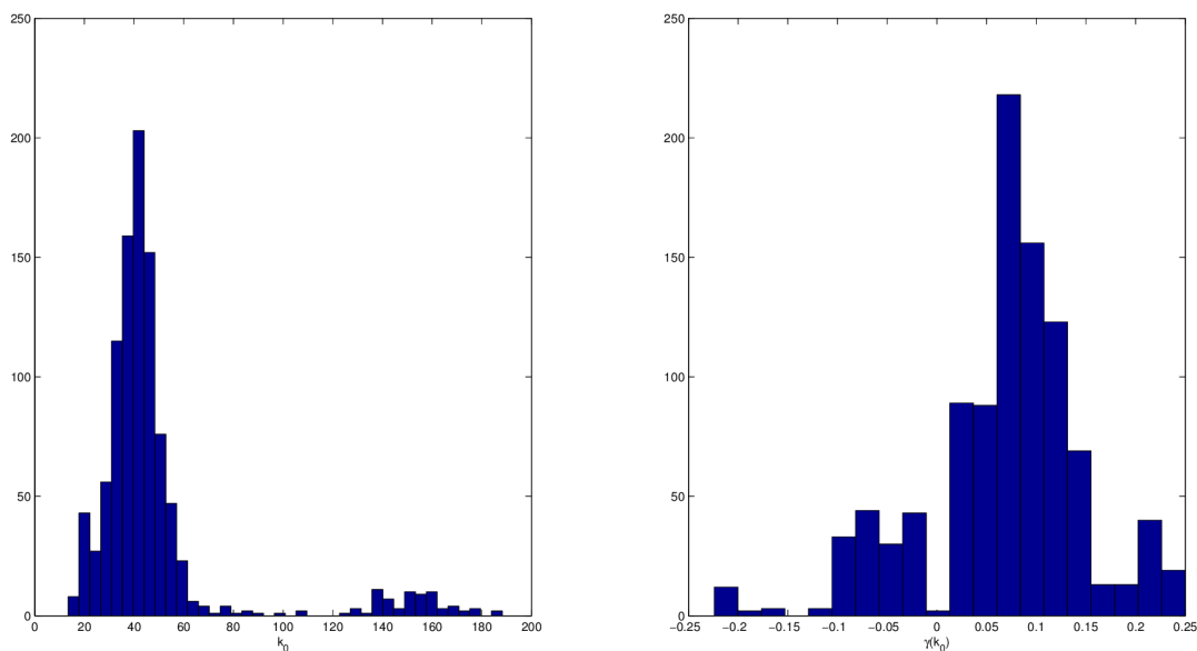
Obrázek 6.11: Histogramy odhadů \hat{k}_0 (vlevo) a \hat{\gamma}_M(\hat{k}_0) (vpravo).
