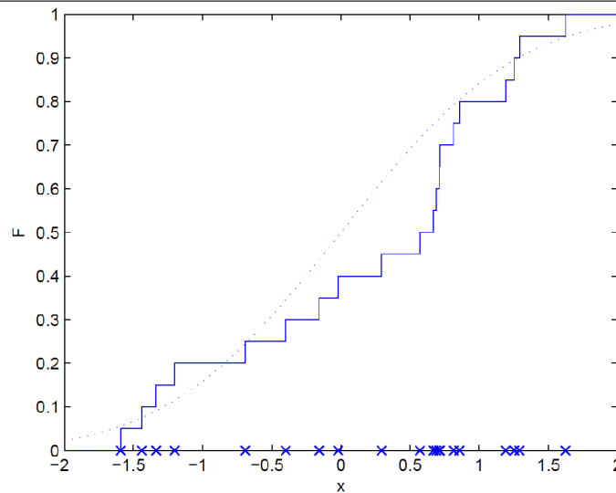
Obrázek 2.2: Empirická distribuční funkce \hat{F}_{20}(x) na základě dvaceti pozorování z normálního rozdělení N(0, 1) . Tečkovaná čára značí skutečnou distribuční funkci F . Realizace náhodného výběru je znázorněna pomocí symbolu \times .
