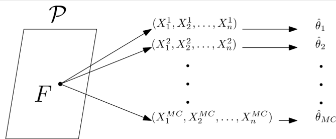
Obrázek 4.1: Schéma Monte Carlo
