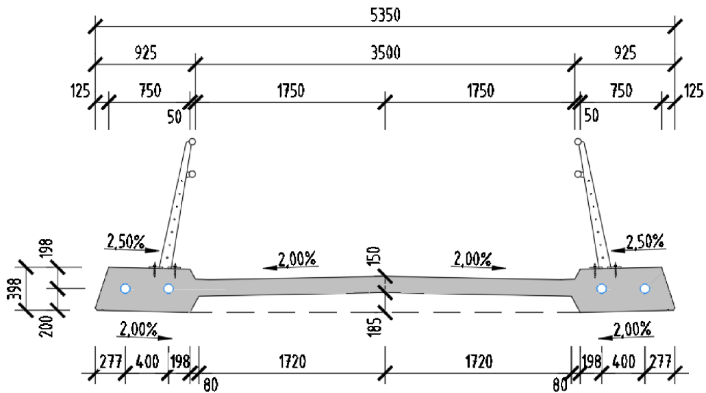
Obrázok 11 Priečný rez – pole
