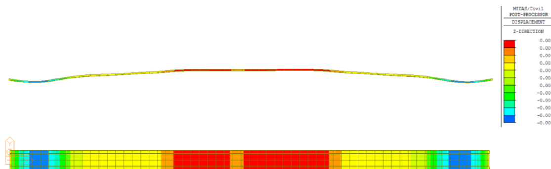
Obrázok 19 Priebeh zvislej deformácie mostovky po vyrovnani
