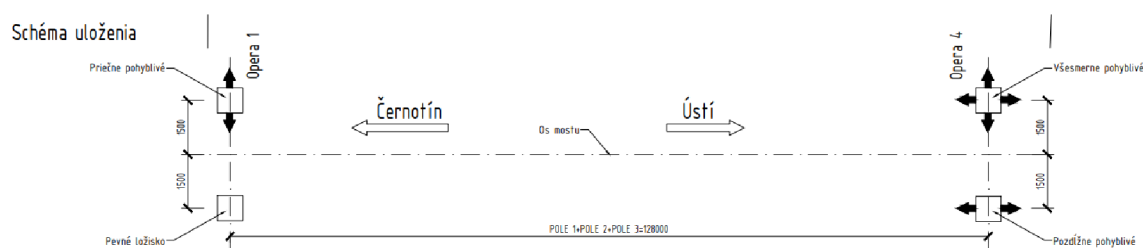
Obrázok 10 Schéma uloženia
