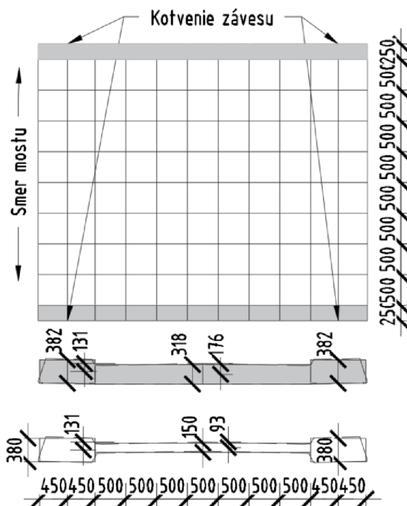
Obrázok 25 Schéma veľkosti elementov – doskostenový model
