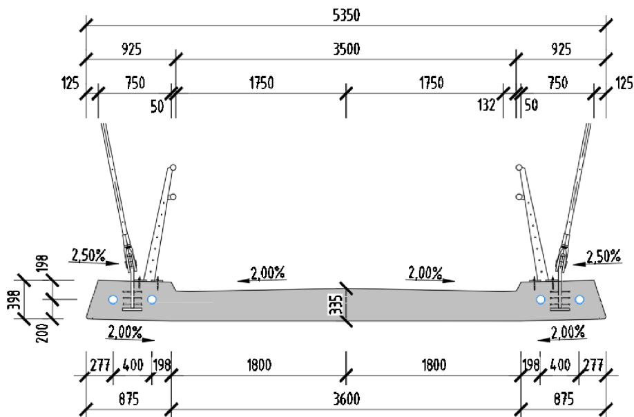
Obrázok 11 Priečný rez – pole
