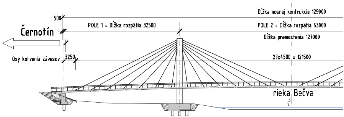
Obrázok 13 Pozdĺžny rez
