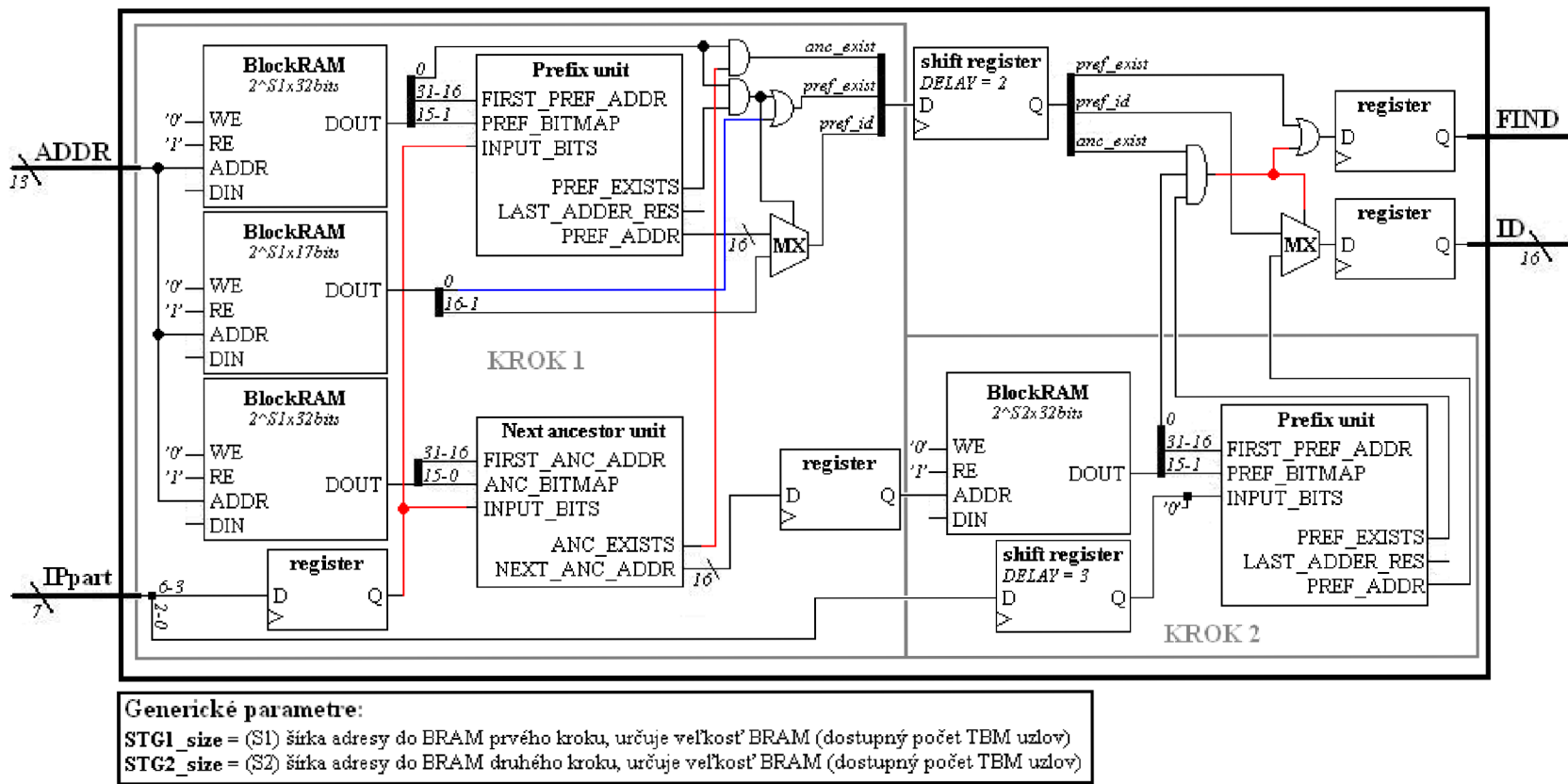
Obr. B.4: Podrobná schéma TBM bloku (dokončenia prefixov)
