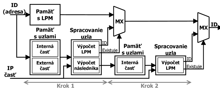
Obr. 4.6: Logická schéma implementácie TBM bloku
