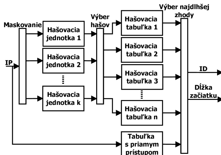
Obr. 4.5: Logická schéma implementácie IP bloku
