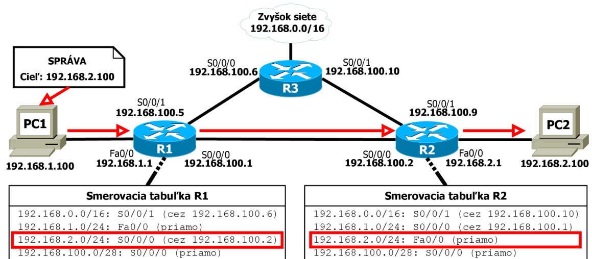
Obr. 2.4: Schéma smerovania správy sieťou
