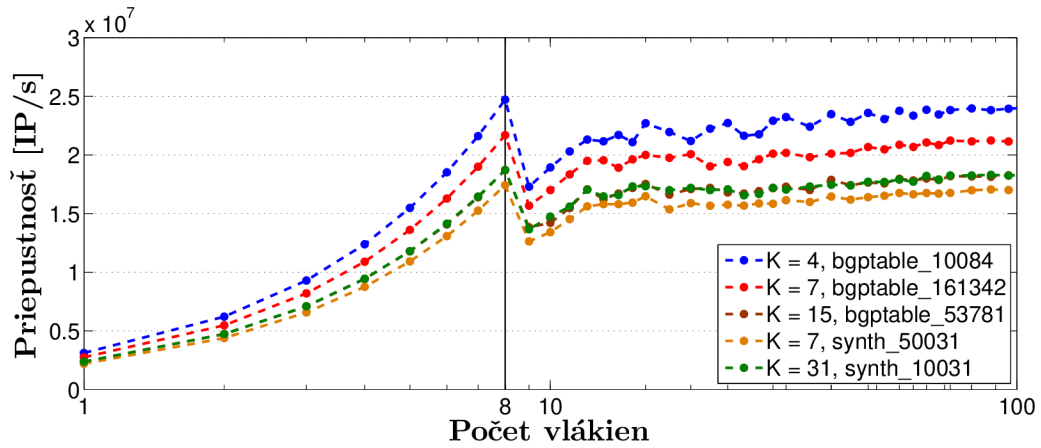
Obr. 5.4: Graf závislosti priepustnosti SST na počte vlákien
