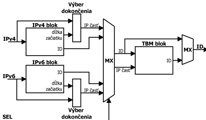
Obr. 4.4: Logická schéma implementácie HW architektúry
