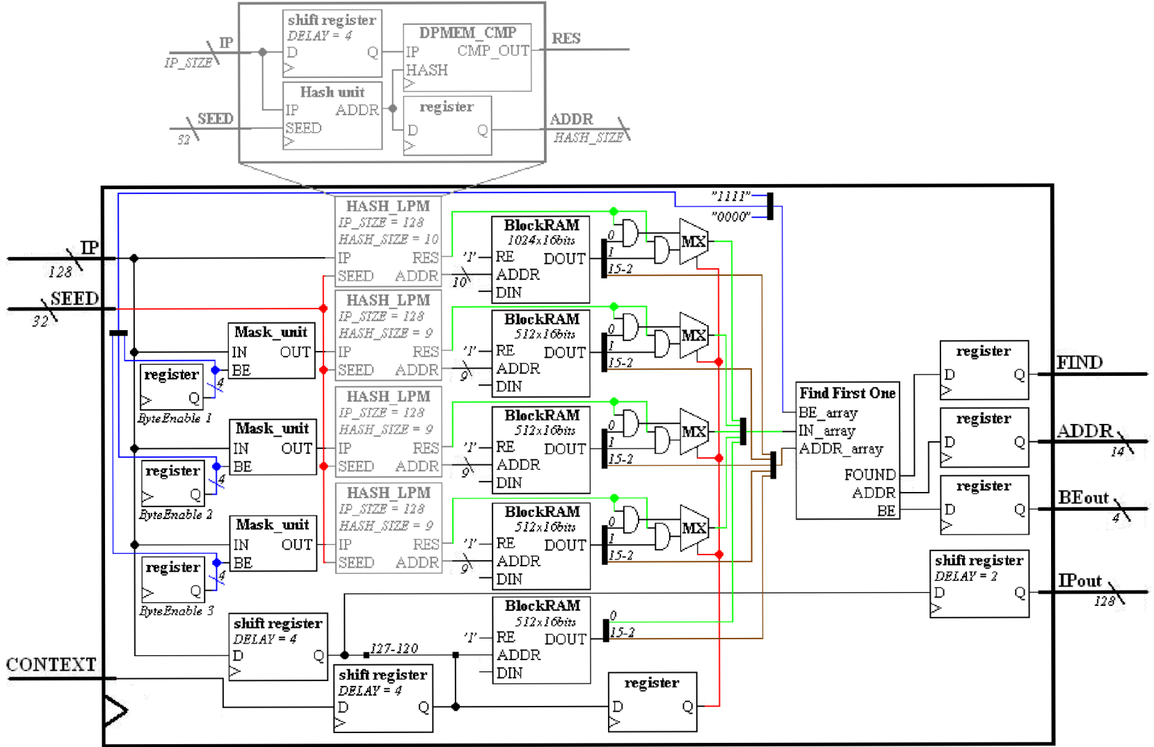
Obr. B.3: Podrobná schéma IPv6 bloku (začiatky IPv6 prefixov)
