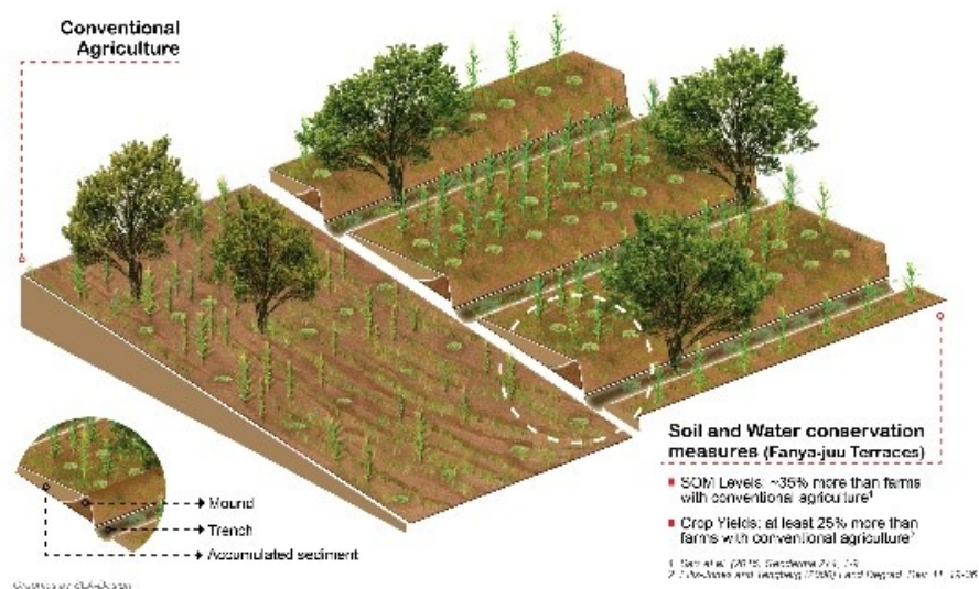
Obrázek 4 Terasování (ccafs.cgiar.org)
