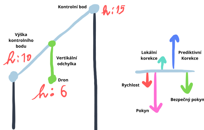
Obrázek 3.9: Pohled z boku - zobrazuje výšku; vpravo pak jsou síly vizualizující vertikální korekci.
