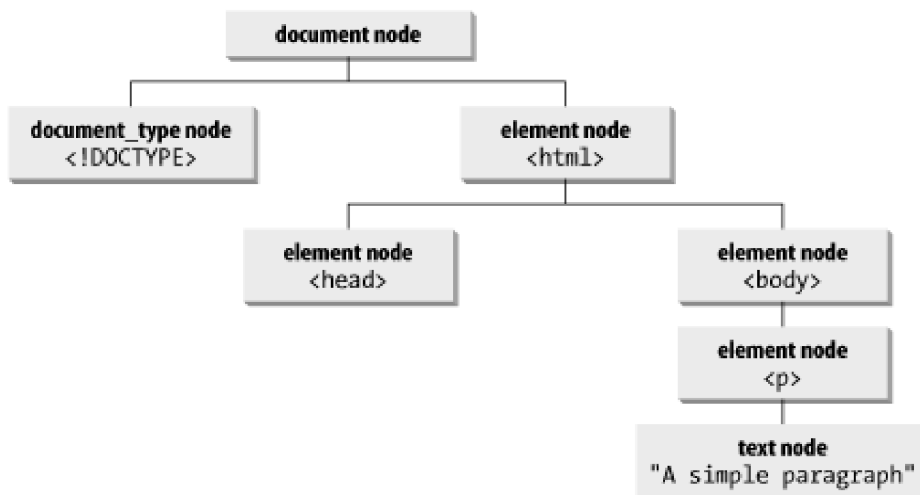
Obrázok 2.2: Hierarchická stromová štruktúra modelu DOM 6
