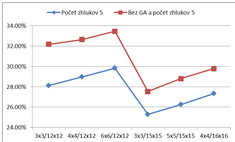
Obr. 6.2: Zníženie počtu porovnávacích operácií použitím GA.
