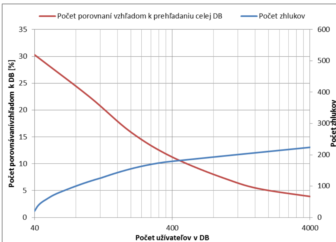
Obr. 4.7: Graf zmeny počtu zhlukov a potrebných porovnávacích operácií vzhľadom k prehľadaniu celej databázy s rastúcim počtom užívateľov v databázy.
