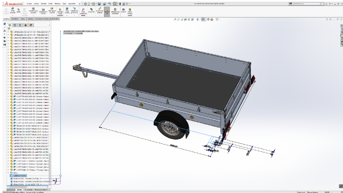
Obrázek č. 13 Pohled na hotový model vozíku pro přípravu automatického generování (Zdroj: Vlastní zpracování)
