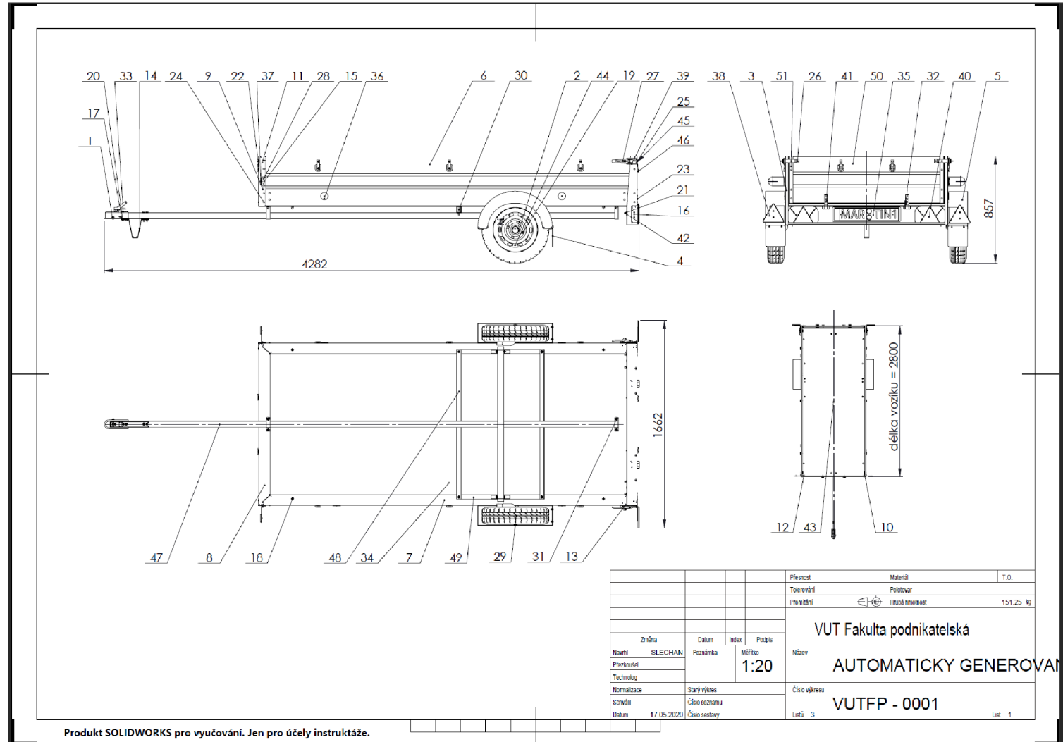
Příloha III Automaticky vygenerovaný výkres přívěsného vozíku (Zdroj: Vlastní zpracování)
