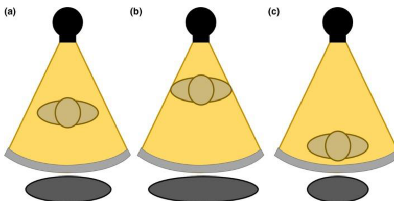
Obrázek 3: Velikost pacienta reprezentovaná rentgenovým snímkem lokalizátoru v důsledku zvětšení, když je pacient (a) vycentrován v gantry, (b) posunut dopředu od středu a (c) posunut dozadu od středu.
