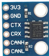
Obrázek 3.6: Budič SN65HVD230 [13]
