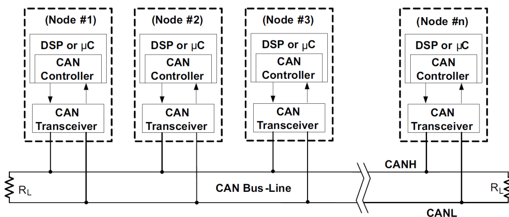
Obrázek 3.1: Struktura uzlů [8]
