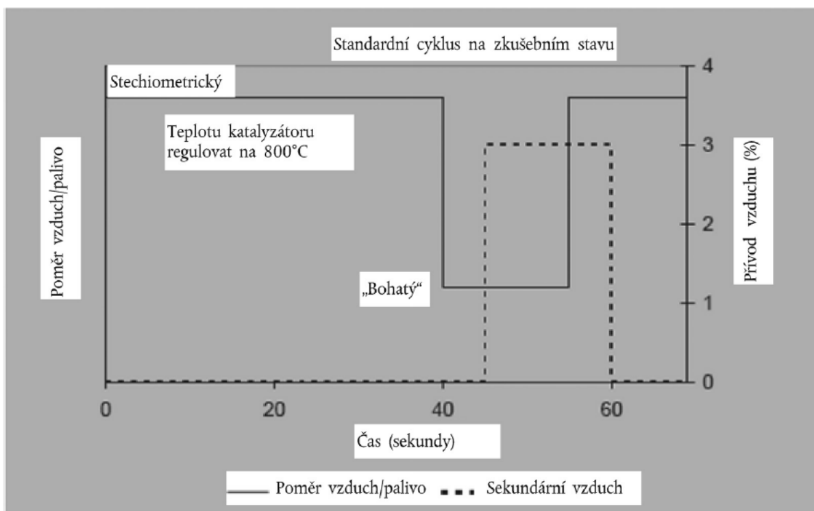
Obr. 2-5 Standardní cyklus na zkušebním stavu [6]
