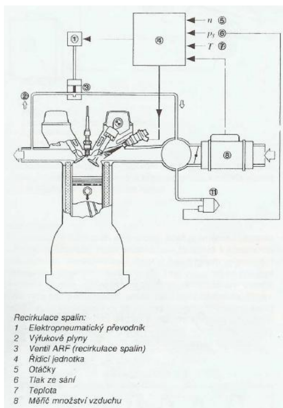
Obr. 4-7 Recirkulace spalin [5]
