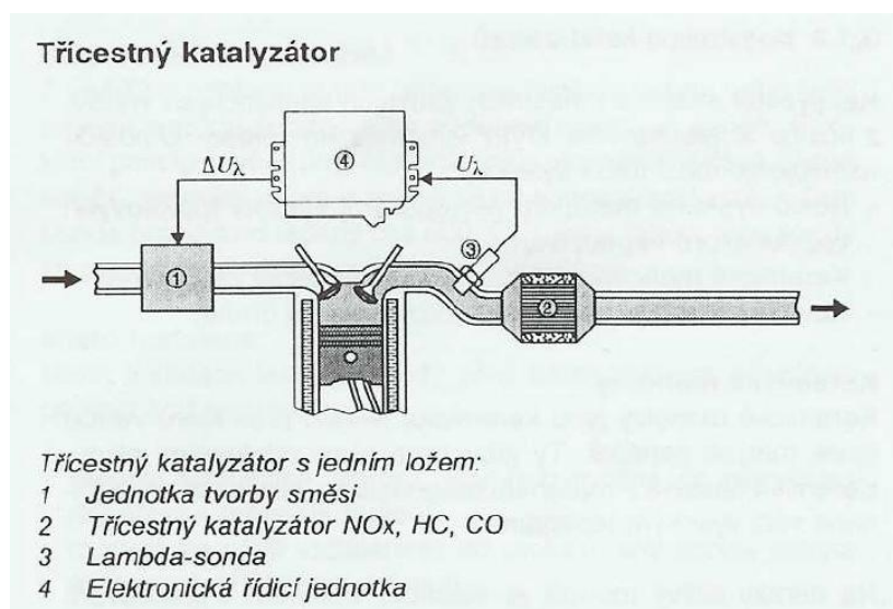
Obr. 4-4 Třícestný katalyzátor s jedním ložem [5]
