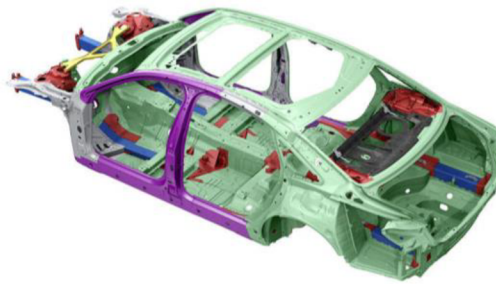
Obrázek 29 Samonosná karoserie
