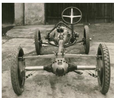
Obrázek 7 Podvozek Tatra 11
