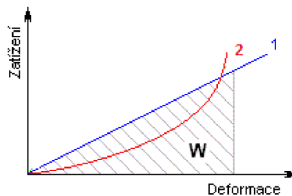
Obrázek 45 Graf porovnání pružin s lineární a progresivní charakteristikou
