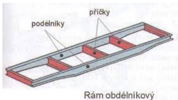
Obrázek 23 Obdélníkový rám
