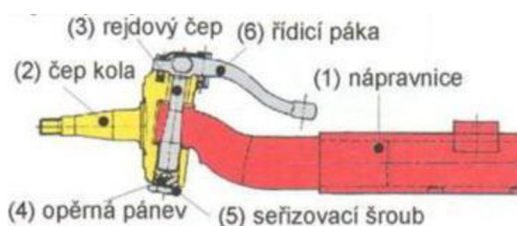
Obrázek 32 Nerozvidlená přední náprava
