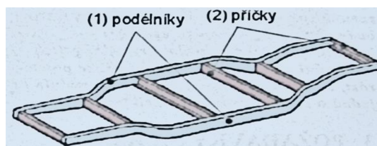
Obrázek 27 Obvodový rám
