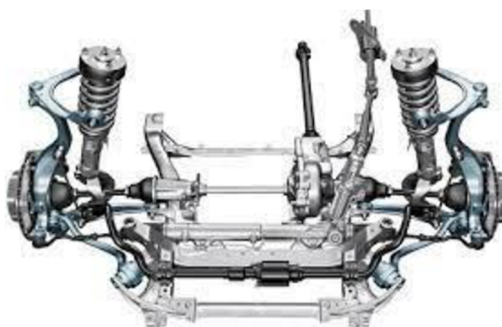
Obrázek 37 Lichoběžníková náprava
