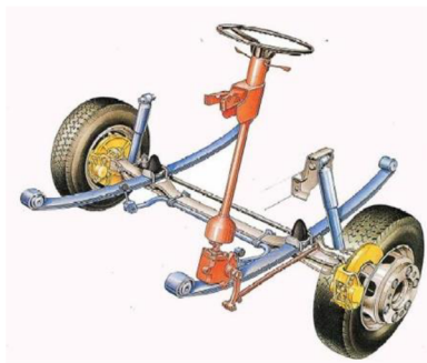
Obrázek 31 Přední tuhá náprava
