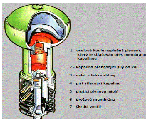
Obrázek 48 Hydropneumatická pružina
