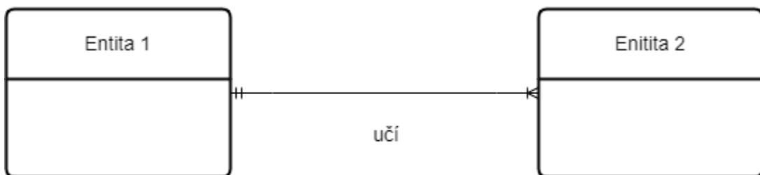
Obrázok č. 15: Prvý typ relácie 1:M zobrazený notáciou Crow's Foot (Zdroj: Vlastné spracovanie podľa (8))
