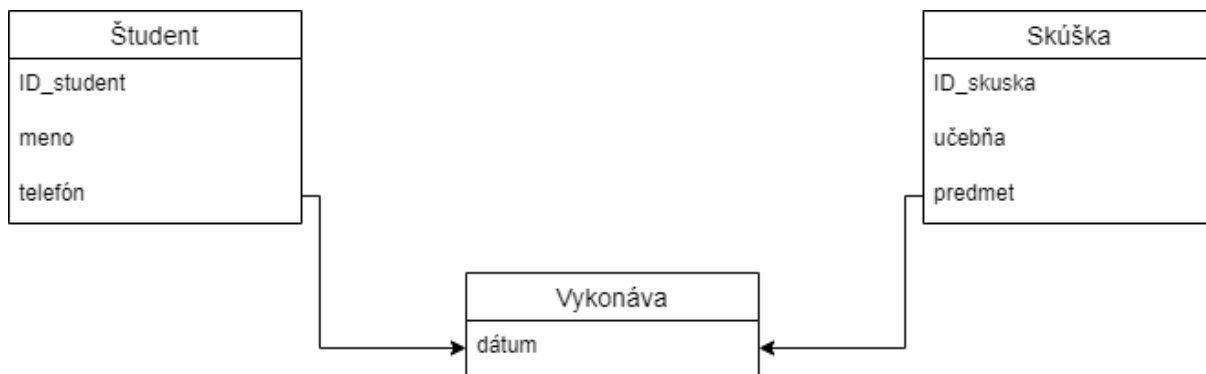
Obrázok č. 8: Schéma sieťovej databázy (vlastné spracovanie podľa (6 s. 11))
