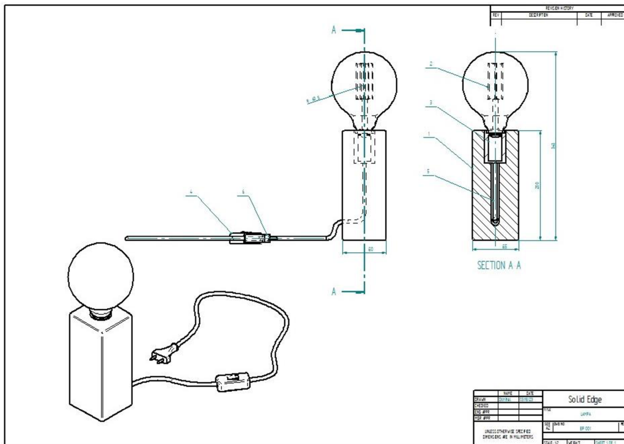
Obrázek 4: Technologický výkres lampy (Zdroj: vlastní zpracování)
